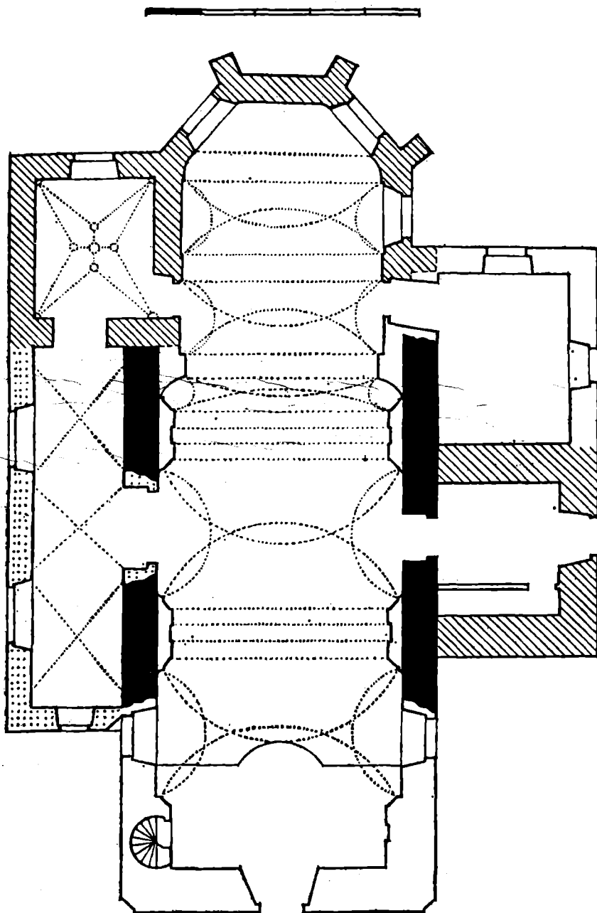
I. Urbanov, kostel sv. Jana Křtitele, půdorys s plně položeným zdivem pozdně románské lodi
