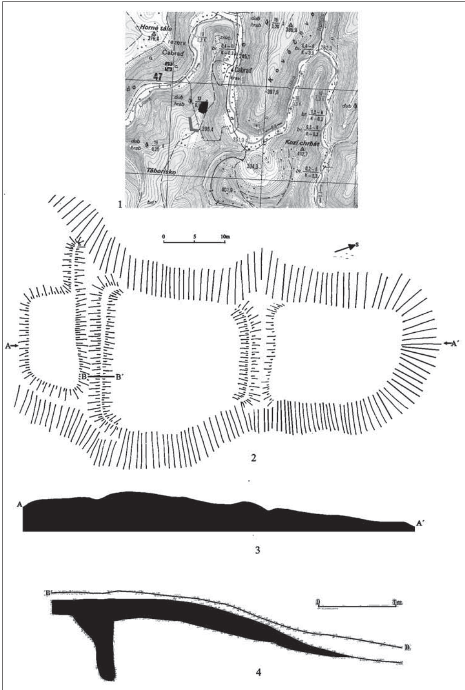
Obr. 2. Zameranie lokality Táborisko. 1 – poloha lokality; 2 – pôdorys ľahkej fortifikácie; 3 – rez terénom ľahkej fortifikácie; 4 – rez fortifikačnými prvками: biela – lesný humus, sivá – obranný násyp, čierna – kolová jama palisády. Kresba M. Miňo. Abb. 2. Ausrichtung der Fundstelle Táborisko. 1 – Lage der Fundstelle; 2 – Grundriss der leichten Fortifikation; 3 – Geländeschnitt der leichten Fortifikation; 4 – Schnitt durch die Fortifikationselemente: weiß – Waldhumus, grau – Verteidigungswall, schwarz – Pfostengrube der Palisade. Zeichnung M. Miňo.
