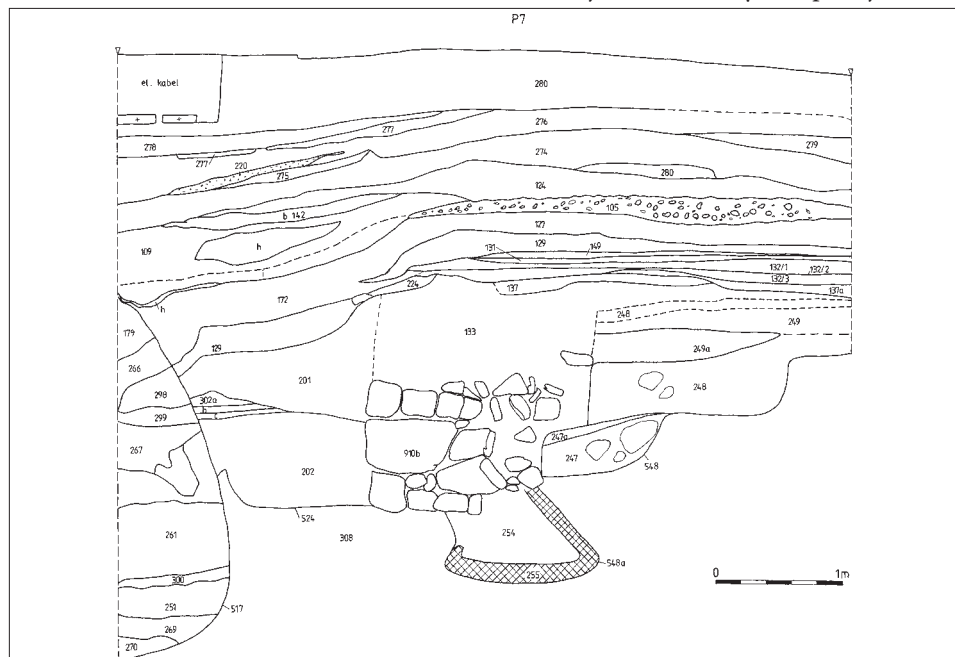
Obr. 13. Josefská 8. Profil při uliční čáře. Jáma 524 se zdí 910b – pyrotechnologické výrobní zařízení porušující pec v jámě 548–548a, obě z první poloviny 13. století; 131, 132/1–3, 1249, 137, 137a – podlahové úpravy povrchového domu, přelom 13. a 14. století; výše souhrn hlinitých a šterkových vrstev 14. století; 517 – obilnice, 14. století. Archiv Archaia Brno, o. p. s., Procházka 1996.
