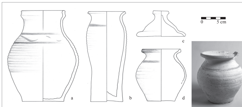
Obr. 13. Praha 1 – Malá Strana. Tvarové spektrum nádob z hrnčířské pece ve Vlašské ulici. Kresba V. Čermák, foto Fr. Malý. Abb. 13. Prag 1 – Kleinsite. Formenspektrum der GefäÙe aus dem Töpferofen in der Vlašská-StraÙe. Zeichnung V. Čermák, Foto Fr. Malý.
