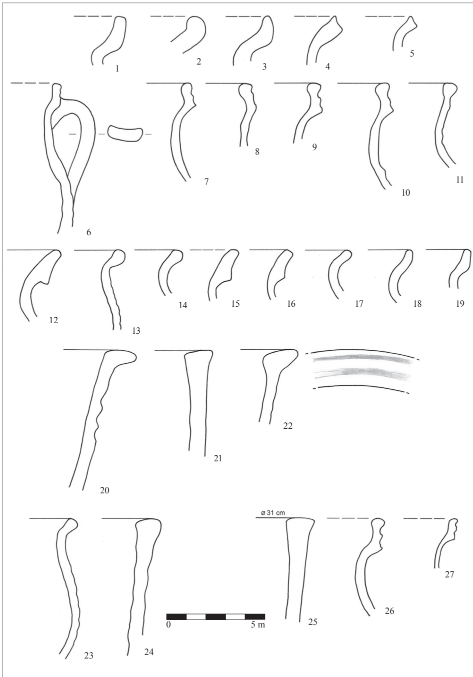
Obr. 7. Praha 1 – Malá Strana, Vlašská ul. čp. 355/III. Kresební dokumentace okrajové profilace nádob z výplně hrnčířské pece (objekt v-04). Kresba V. Čermák.
