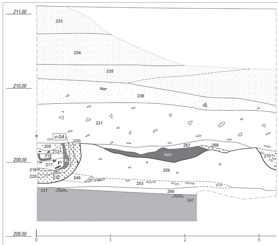
Obr. 6. Praha 1 – Malá Strana. Řez R11 v sondě II. Západně od pece v-04 byla odkryta mělká jáma (deponie hrnčířské suroviny) vyplněná jílovitou hlinou (vrstva 266 – tmavě šedě). Kresba J. Hlavatý. Abb. 6. Prag 1 – Kleinsseite. Schnitt R11 in Sondagrabung II. Westlich von Ofen v-04 wurde eine flache Grube freigelegt (Töpferrohstoffdeponie), die mit tonartigem Lehm verfüllt war (Schicht 266 – dunkelgrau). Zeichnung J. Hlavatý.
