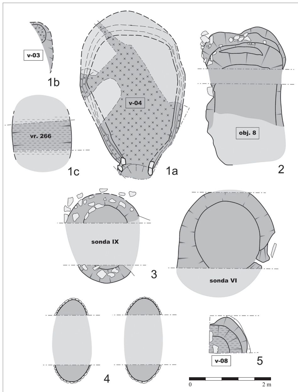
Obr. 17. Pece a další objekty spojené s hrnčířskou výrobou z vrcholně středověké Malé Strany. 1 – objekty z hrnčířské dílny ve Vlašské ul. čp. 355/III: 1a – pec v-04; 1b – pec v-03; 1c – deponie suroviny, jáma s jilem (Havrda–Matějková 2014, půdorys P02 a P03, kresba J. Havrda a J. Hlavatý); 2 – pec západně od Malostranského nám. čp. 258 (Čiháková–Zavřel 1995, 277; Hentsch 2010, obr. 38, kresba J. Vachuda); 3 – pece ve Valdštejnské ul. čp. 162/III (Omelka 1995, půdorys 1 v sondě VI a půdorys 1 v sondě IX, kresba M. Omelka a R. Tvrđík); 4 – pece na západním konci Hellichovy ulice (Huml 1971, kresba St. Pekař); 5 – deponie hrnčířského (?) jilu na nádvoří domu čp. 450 v ul. Újezd (Tryml 2004, kresba J. Vachuda). Grafická úprava půdorysů objektů J. Hlavatý.
