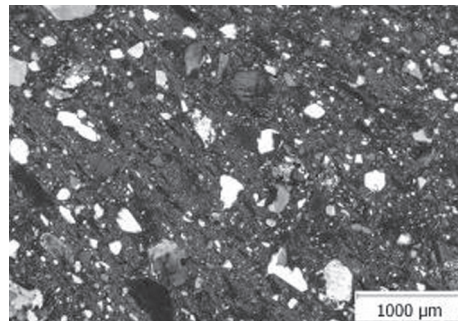
Obr. 20. Výbrus vzorku č. 12539-4 (2. polovina 10.–11. století). Na snímku je patrná orientace střepevé hmoty i uvnitř vzorku, to svědčí o kvalitnějším a rychlejším obtáčení nádoby. Foto A. Kloužková. Abb. 20. Schliff von Probe Nr. 12539-4 (2. Hälfte 10.–11. Jhd.). Auf der Aufnahme ist die Orientierung der Scherbenmasse auch im Innern der Probe erkennbar, das deutet auf eine qualitativ bessere und schnellere Drehung des Gefäßes hin. Foto A. Kloužková.
