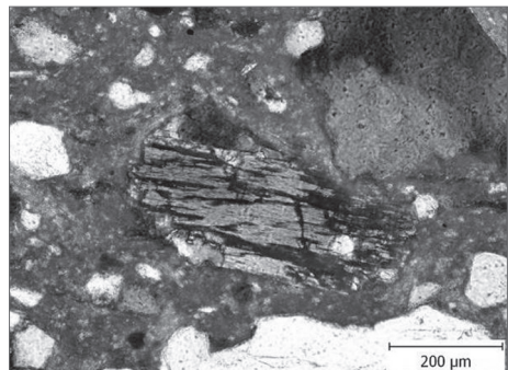
Obr. 12. Výbrus vzorku inv. č. 12539-4 (2. polovina 10.–11. století). Na snímku uprostřed zrně hornblendu (XL). Foto A. Kloužková. Abb. 12. Schliff von Probe Inv.-Nr. 12539-4 (2. Hälfte 10.–11. Jhdt.). In der Mitte der Aufnahme ein Hornblendekorn (XL). Foto A. Kloužková.
