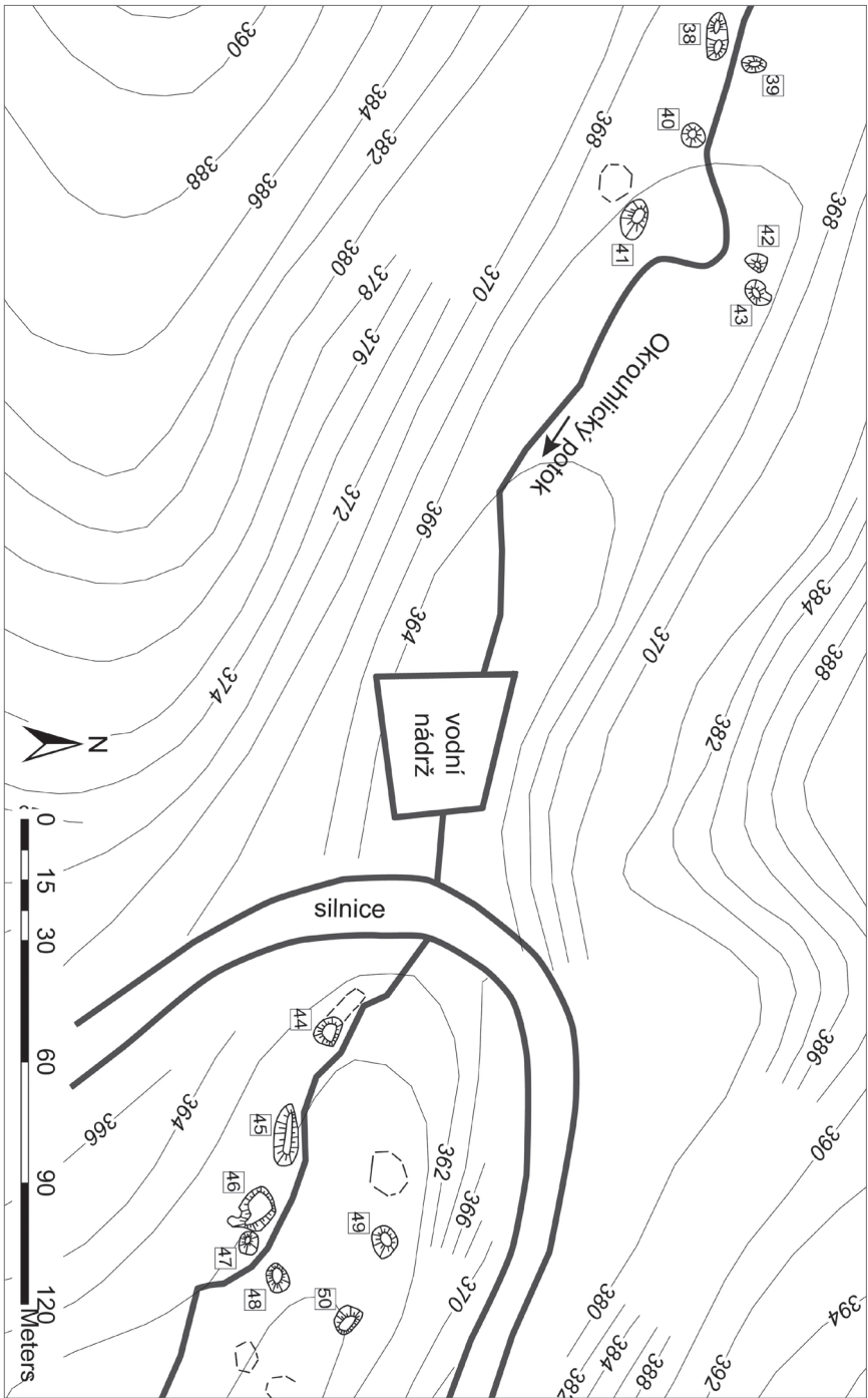
Obr. 4. Zamerění reliktů po těžbě zlata na rýžovišti B. Půdorysný plán 3. Abb. 4. Vermessung der Goldgewinnungssprekire an Seitenlagerstätte B. Grundrissplan 3.
