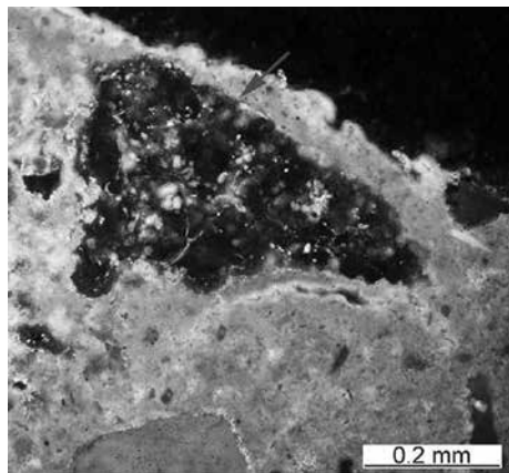
Obr. 4. Fragments sklářské strusky na výbrusu vzorku JK. Foto D. Všíanský.
