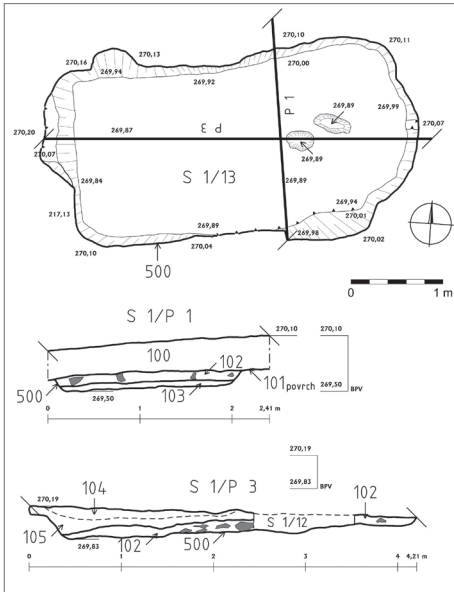
Obr. 9. Haňovice. Půdorys odkrytého objektu. Kresba K. Faltýnek. Abb. 9. Haňovice. Grundriss des freigelegten Objektes. Zeichnung K. Faltýnek.
