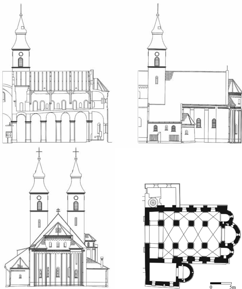
Obr. 5. Diakovce, niekdajší kláštorň Kostol Panny Márie, súčasný stav – pôdorys, pozdĺžny severný rezopohľad, južný a východný pohľad. Podklady Archív Pamiatkového úradu SR, Zbierka projektov a plánov, sign. A7478.
