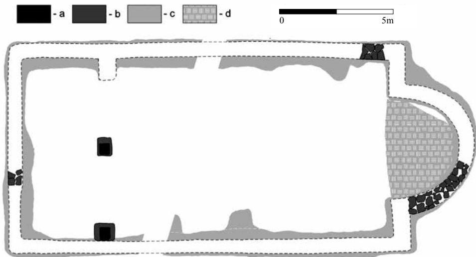
Obr. 21. Biňa, poloha Opátske, zaniknutý kostol v mieste zaniknutej stredovekej dediny. a – nadzákladové murivo, b – základy, c – základová ryha, d – dlážka. Podľa Pomfyová–Samuel–Žažová 2014 na základe nepublikovaných archívnych materiálov A. Habovštiaka. Abb. 21. Biňa, Lage Opátske, untergegangene Kirche an der Stelle einer mittelalterlichen Dorfwüstung. a – Mauerwerk über dem Fundament, b – Fundament, c – Fundamentrinne, d – Fußboden. Nach Pomfyová–Samuel–Žažová 2014 auf Grundlage unveröffentlichten Archivmaterials von A. Habovštiak.
