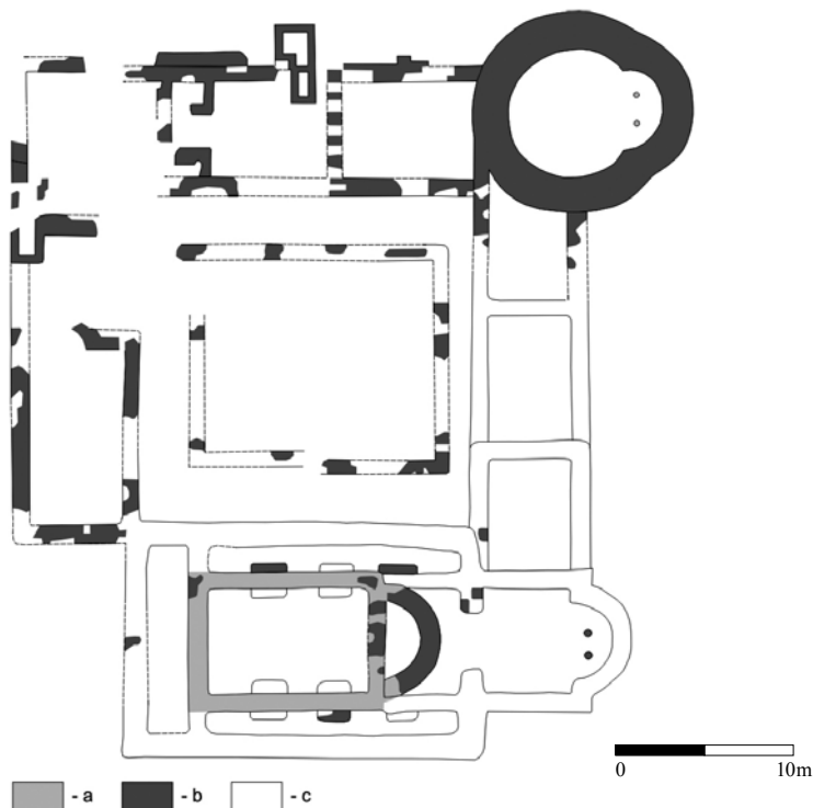
Obr. 12. Krásna nad Hornádcom, pôdorys pôvodného kostola (a), trojlodového kláštorného kostola a vnútornej klauzúry. a, c – základové ryhy, b – zachované, prevažne základové murivá.
