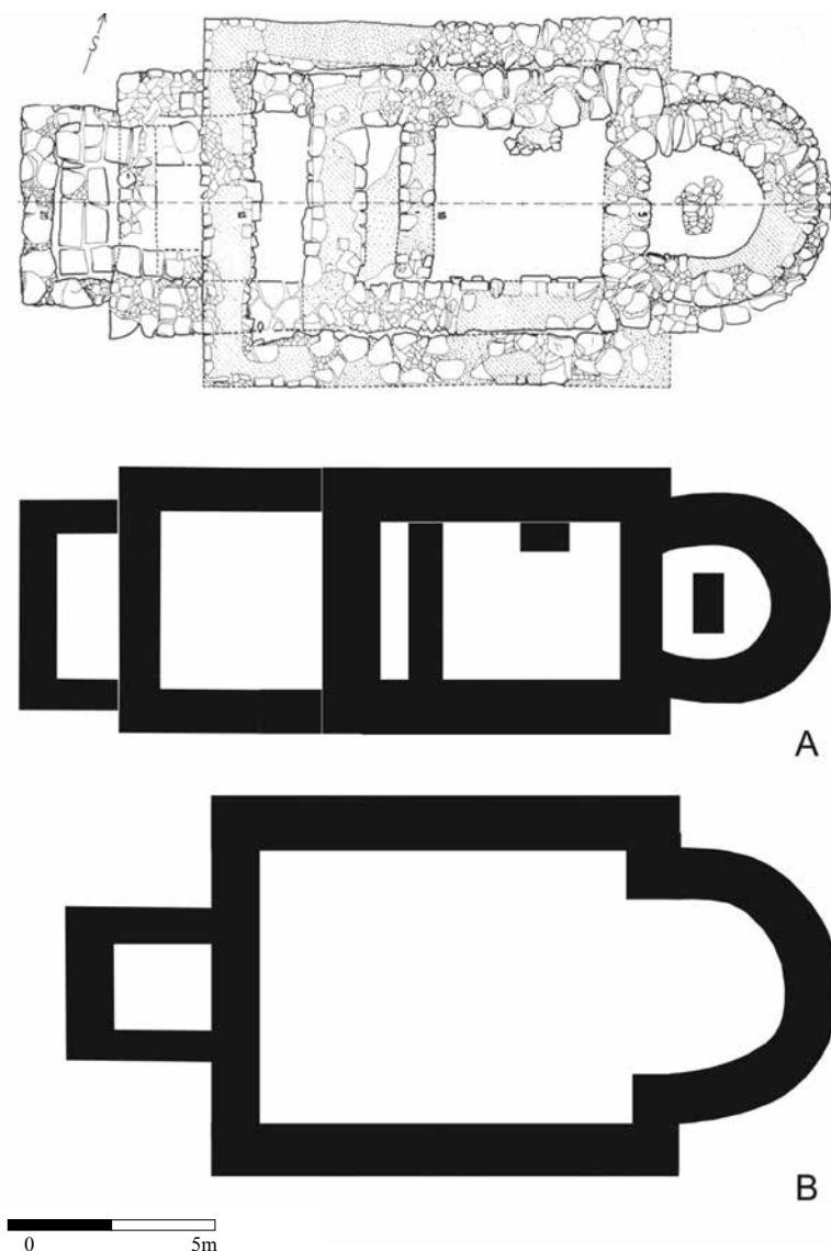
Obr. 22. Levice, poloha Bratka, zaniknutý kostol v mieste zaniknutej stredovekej dediny, superpozícia staršej (A) a mladšej (B) stavby a ich jednotlivé pôdorysy. Podľa Habovštiak 1963a.
