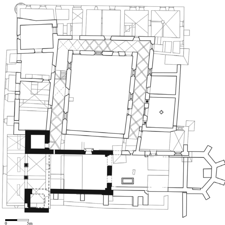
Obr. 7. Bzovík, zaniknutý premonštrátsky (pôvodne benediktínsky) kláštor, pôdorys kostola a vnútornej klauzúry s vyznačením románskych murív kostola. Podľa Mencl 1937.
