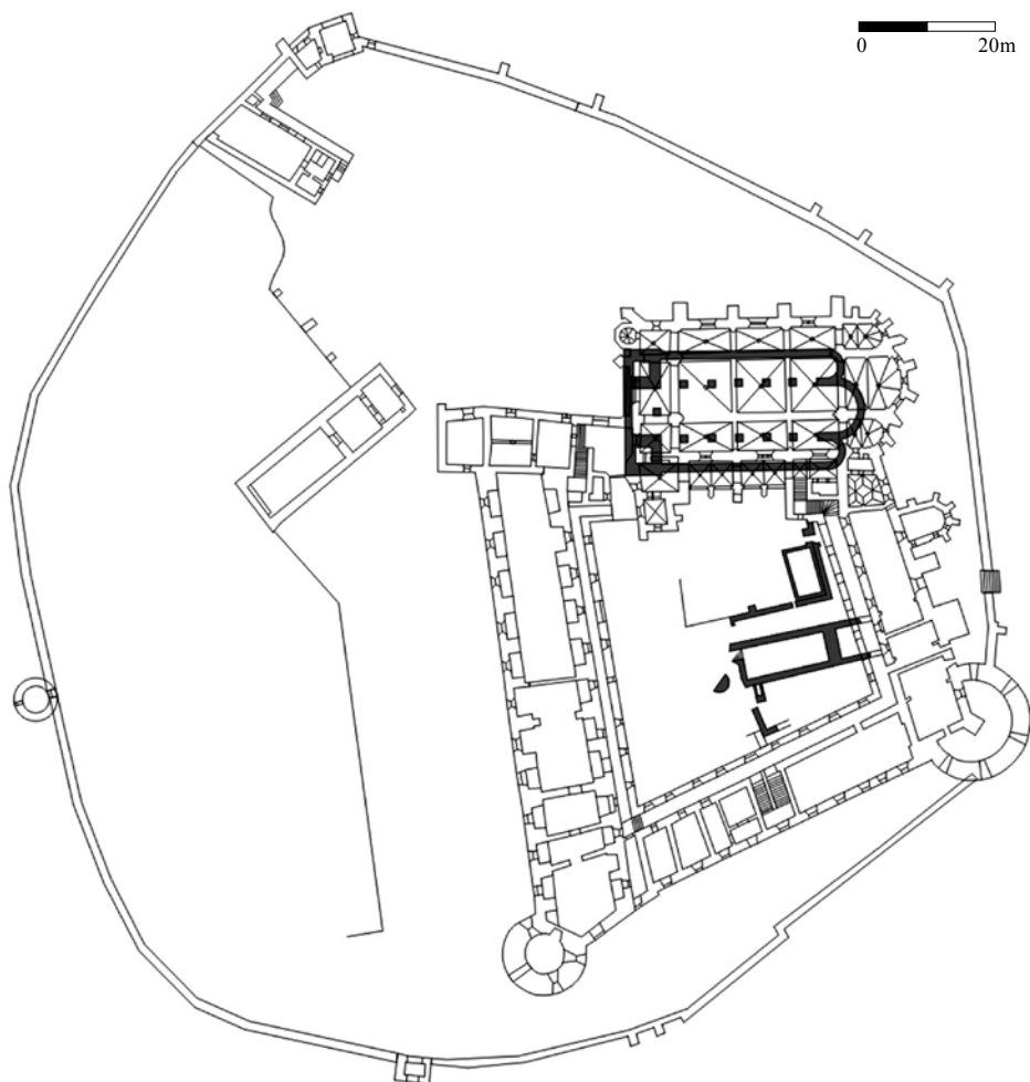
Obr. 4. Hronský Beňadik, areál niekdajšieho benediktínskeho kláštora s vyznačením pôdorysu zaniknutého románskeho kostola (ideálna rekonštrukcia podľa F. Knauza [1890]) a archeologicky odkrytých častí vnútornej klauzúry. Podľa Habovštiak–Holčík 1994. Abb. 4. Hronský Beňadik, Areal des ehemaligen Benediktinerklosters mit eingezeichnetem Grundriss der untergegangenen romanischen Kirche. Ideale Rekonstruktion nach N. Knauz (1890) und archäologisch freigelegte Teile der inneren Klausur. Nach Habovštiak–Holčík 1994.
