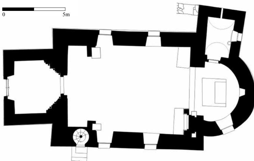
Obr. 31. Ilija, Kostol sv. Egídia. Zameranie Oddelenie grafickej dokumentácie Pamiatkového úradu SR, doplnené podľa Labuda-Paulusová 2003.
