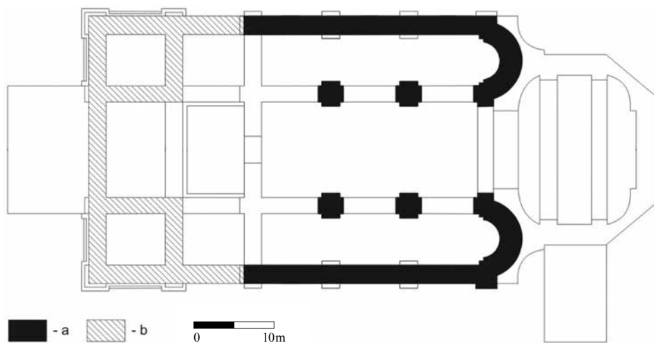
Obr. 18. Hronovce-Čajakovo, niekdajší benediktínsky kláštorňý kostol. a – stojace románske murivá, b – zaniknuté románske murivá. Podklad Archív Pamiatkového úradu SR, Zbierka schematických zameraní, sign. V 1319.
