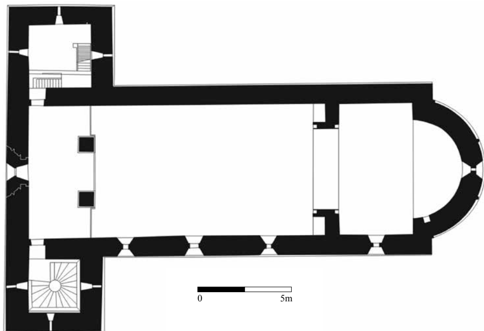
Obr. 9. Rimavské Janovce, pôdorys niekdajšieho kláštorného Kostola sv. Jána Krstiteľa. Zameranie Oddelenie grafickej dokumentácie Pamiatkového úradu SR.
