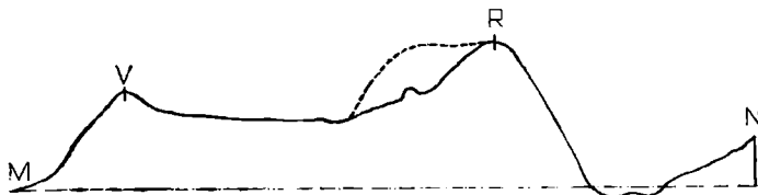
Obr. 6. Profil opevněného objektu na „Horním hrádku“ u Lhotic, okr. Třebíč. (Převýšeno dvaapůlkrát, kresba P. Michna.)
