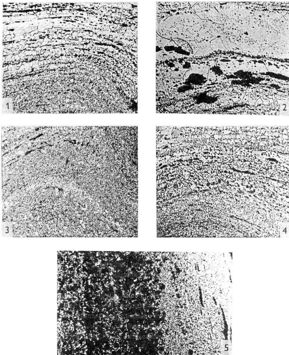
Obr. 2. Mikulčice. Mlat vz. 532. Mikrostruktury po leptání 2% nitalem: 1 — 4 vz. A — zakřivené pásy ferritického železa se stopami perlitu, černě struskové vměstky. 5 vz. B připojená stře-pinka perlitické ocele (tmavě) a ferritické pásy (světle). Zvětšení 50x.
