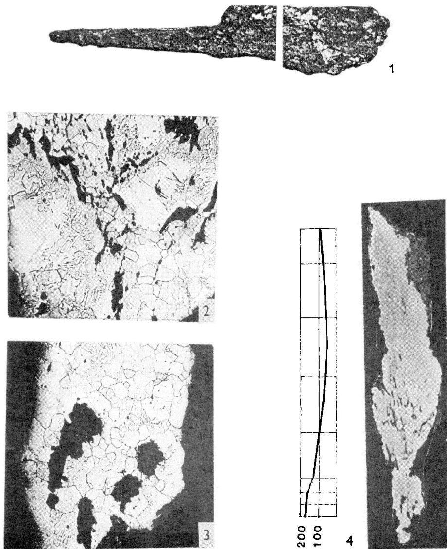
Obr. 4. Mikulčice. Zlomek nože vz. 534.1 nůž se zakresleným odběrem vzorku. 2 ferrit se sva-rem V mezi ostřím a hřbetem. 3 Ferrit a vměstky (tmavě) v břitu. 4 Makrosnímek po leptání 5% nitalem a průběh mikrotvrdomosti mHV 30g. 2 a 3 zvětšení 100x, 4 zvětšení 5x.
