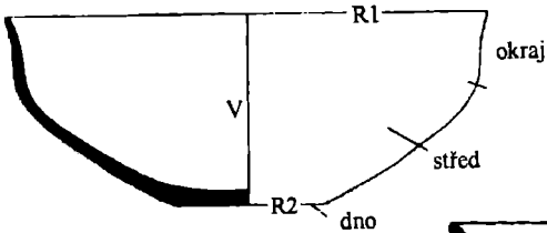
Miska s prohnutým okrajem (miska po)
