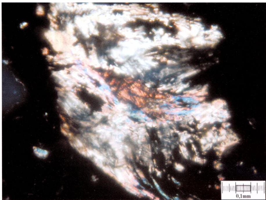
Obr. 1: Těšetice „Sutny“, grafitová keramika HD2, 1686A (100-120), rutil v grafit-sericitové břidlici, XN, 10 \times .
