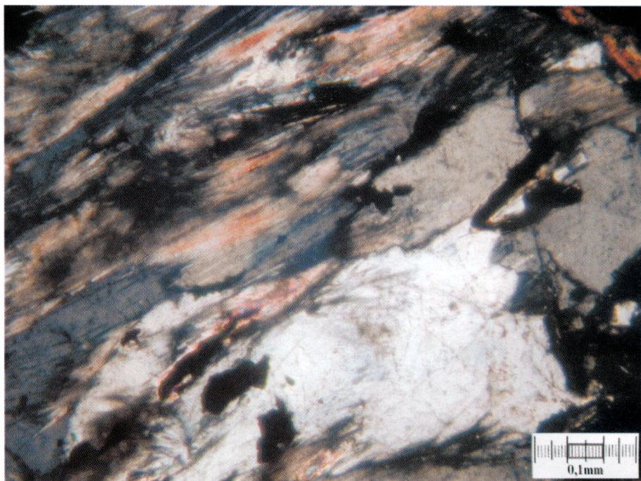
Obr. 5: Těšetice „Sutny“, grafitová keramika HD2, 1640B (60-80), úlomky sillimanitových rul grafitem, XN, 10×
