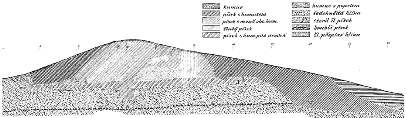
Obr. 223 – Strachotín. Výzkum B. Novotného z roku 1960 (podle Novotný 1963–1964).
