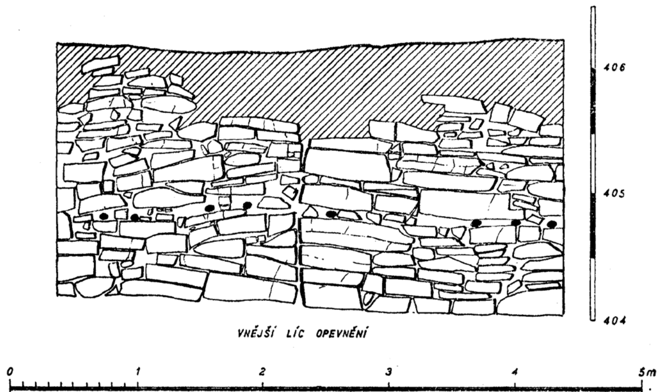
Obr. 230 – Libušín. Čelní pohled na vnější líc hradby. Černá kolečka jsou zuhelnatělé klády roštu (podle Vána 1973a).
