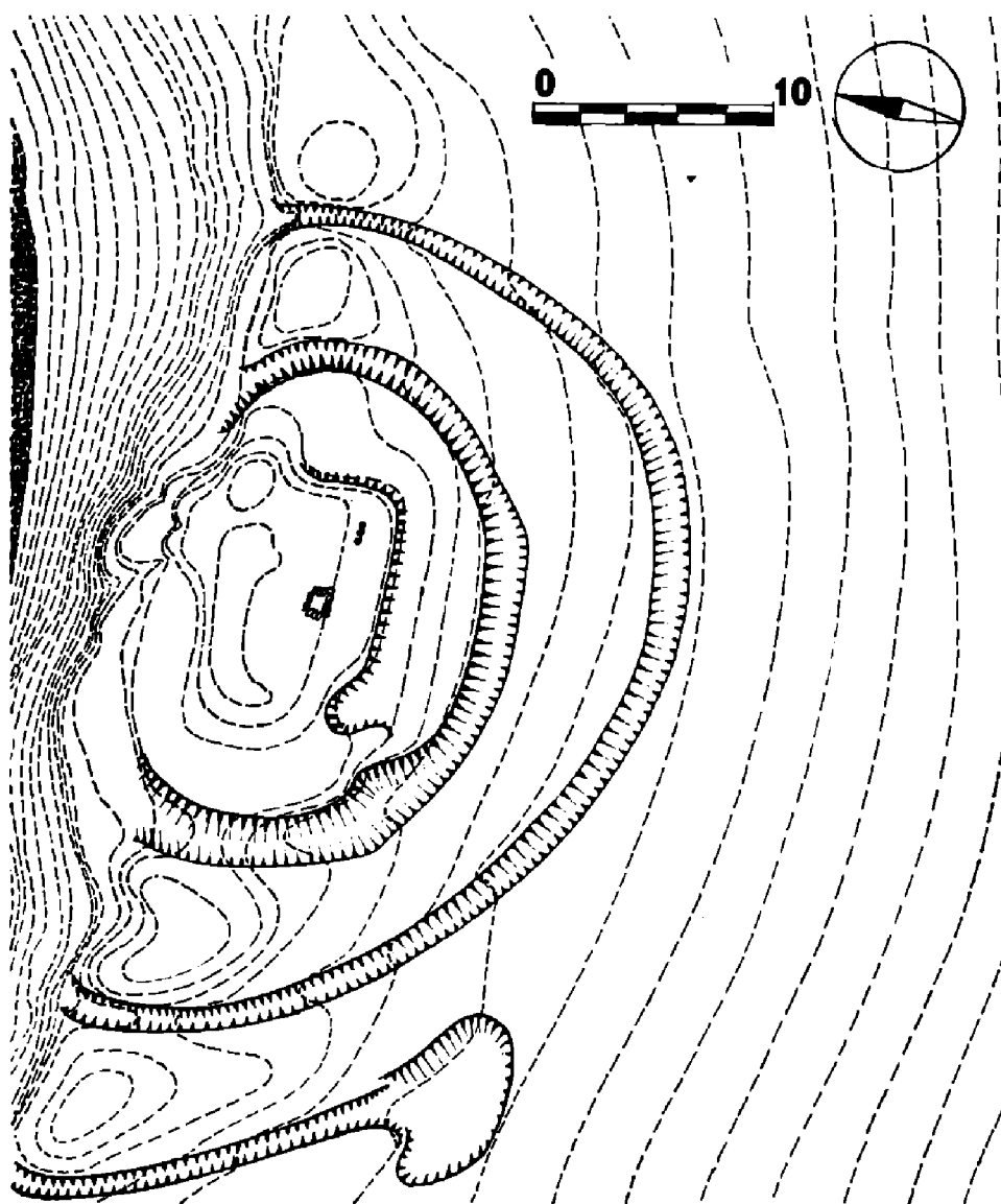
Obr. 5. Schéma fortifikace II.
