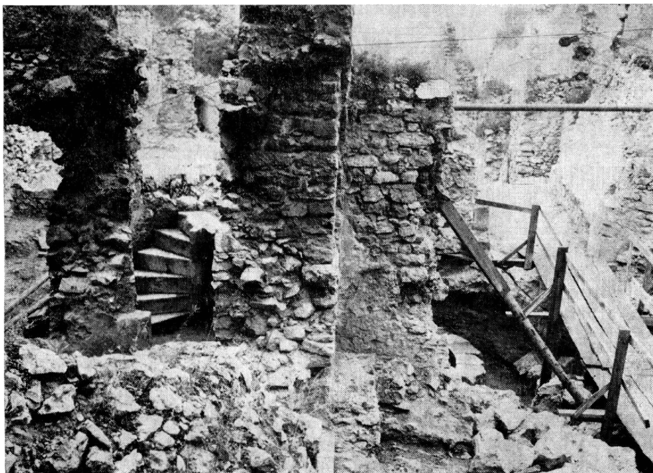
Obr. 5. Beckov, hrad. Pohľad na priečny palác so sediliovou chodbou. Foto D. Tóth.
