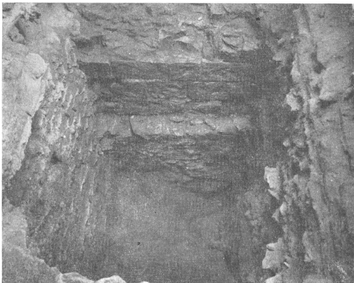
Obr. 3. Praha 1, kostel sv. Martina ve zdi. Vnější líc jižní stěny románského kostela s třemi řádky nadzemního zdiva a s rozšířeným základem. Vlevo cihlové zdivo novověké hrobky. Pohled od jihu. Foto Z. Helfert.
