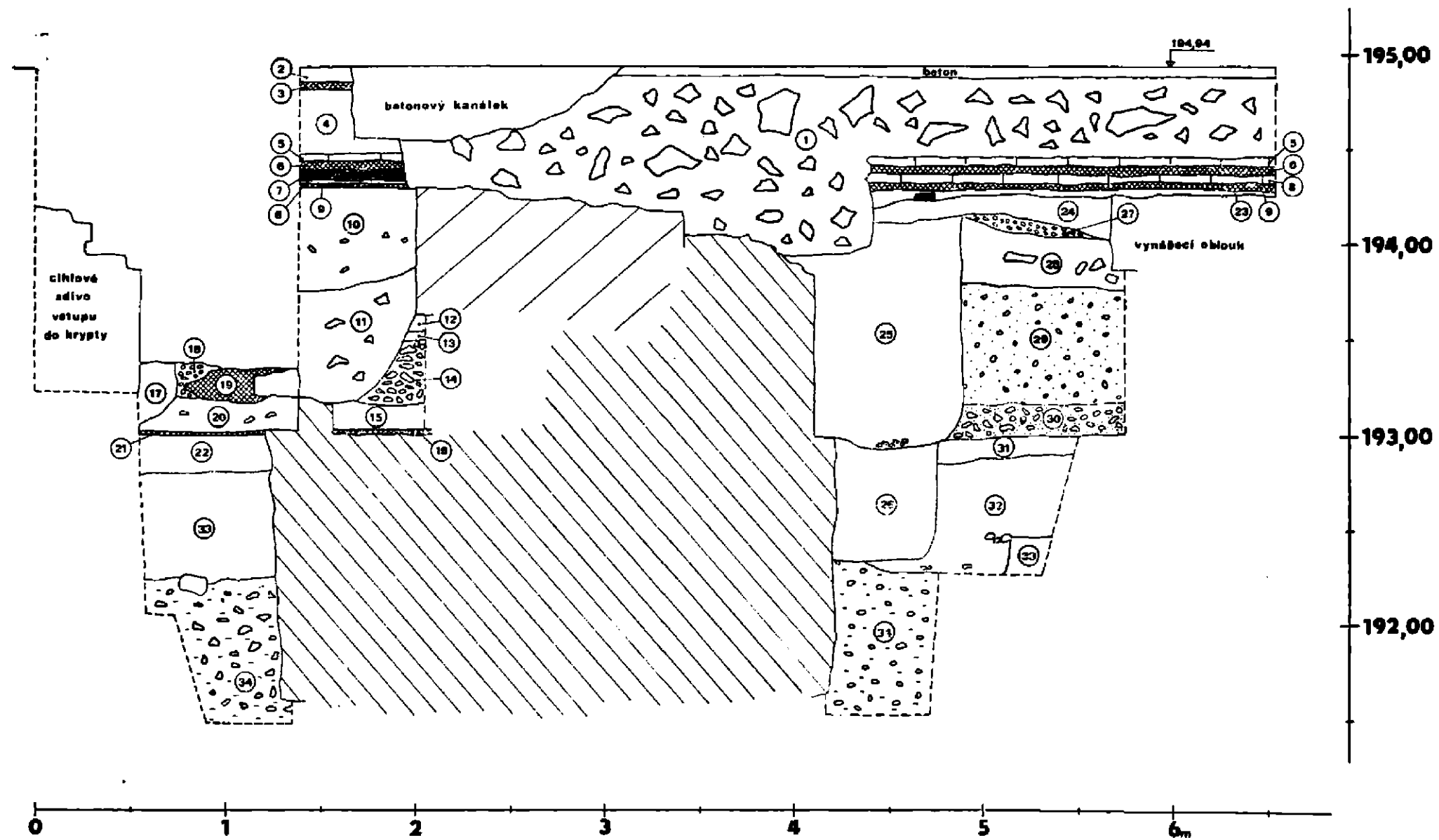
Obr. 1. Praha 1, kostel sv. Martina ve zdi. Východní profil sondy. Hustá šra fura zobrazuje románské, řidší gotické zdivo. Kresba Zd. Dragoun a J. Meurek.
