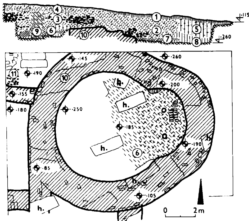
Obr. 3. Košice-Krásna: Plán rotundy s profilom. 1 – mačtinovitá vrstva, 2 – hrubá deštrukcia, 3 – tehlové úlomky, 4 – žltý íl, 5 – íl prelešaný suťou, 6 – vrstva maltoviny 7 – čierna zem, 8 – ílovité podložie, 9 – novoveký zásah, 10 – základové murivo, 11 – vrstva štrku, h – hrobové jamy. Kresba: K. Fűrývová.
