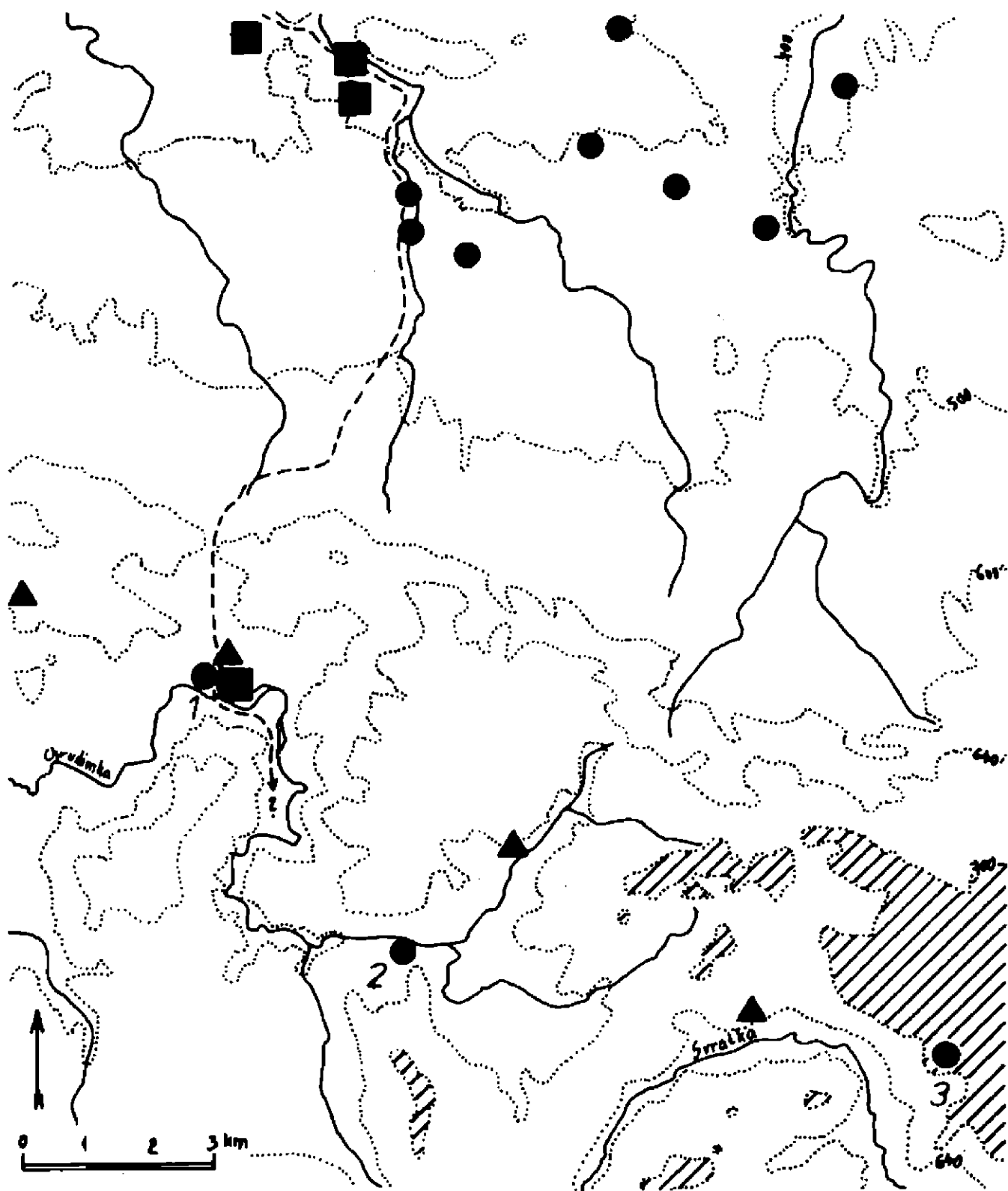
Obr. 4. Hlinsko a přilehlá část Chrudimska. □ - označují osídlení doložené do konce 12. století; ○ - osídlení 13. století; △ - farní kostely doložené k r. 1340-50 (vyznačeno pouze na Hlinsku); --- - trasa předpokládané cesty. Plochy nad 700 m n. m. šrafovány. 1 - Hlinsko, 2 - Lány u Hlinska (k. ú. Kameničky), 3 - Svatouch „Zkamenělý zámek“. Kresba J. Frolík.
