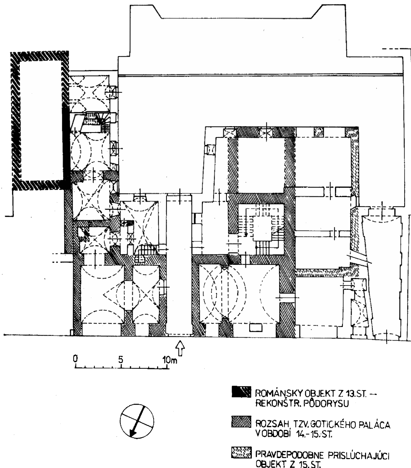
Obr. 1. Bratislava, býv. Pálffyho palác na Nálepkej ul. 19–21. Pôdorys prízemnia s umelecko-historickou analýzou hlavných stredovekých fáz vývoja objektu. Zakreslené do stavu objektu z r. 1979–1982.
