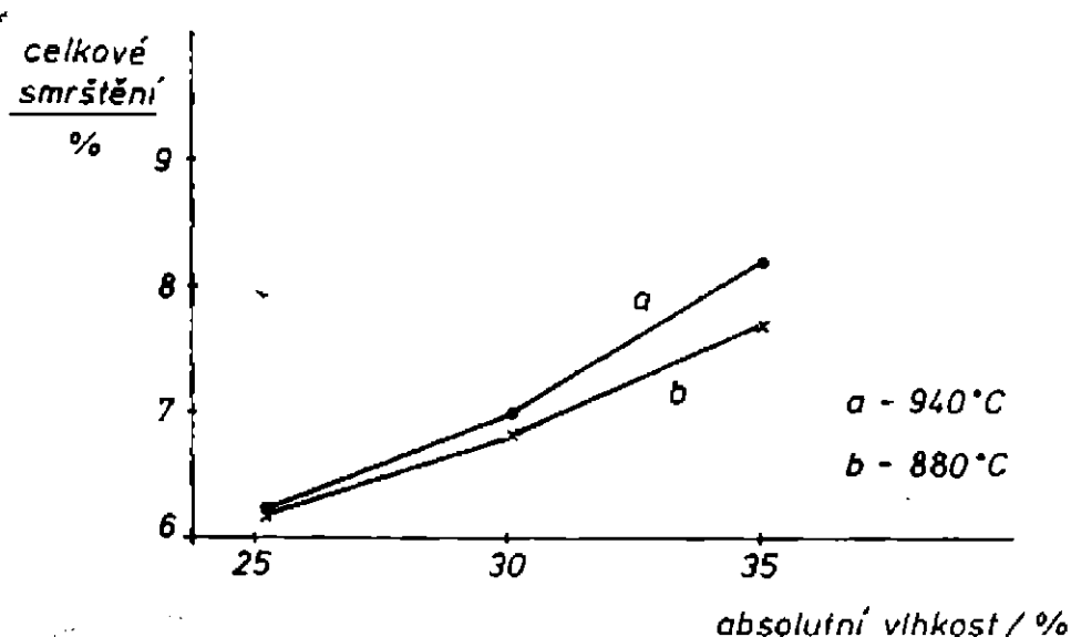
Obr. 2. Závislost celkového smrštění na vytvářecí vlhkosti pro různé teploty výpalu (a=940 °C, b=880 °C) pro směs 70 ‰ Vonšov/30 ‰ písek.
