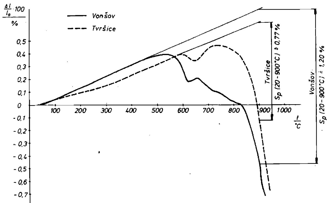
Obr. 1. Křivky DZ čistých jílu Vonšov a Tvršice s orientačním vyhodnocením smrštění pálením ( S_p ) při výpalu na 900 °C.
