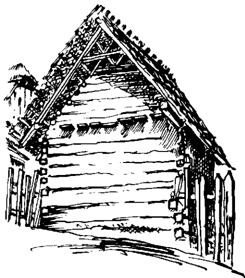
13. Roubená klanba u sýpky, Komenica žp. 108, o. Prešov (podle J. V. Scheybala).
