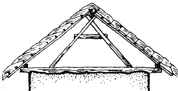
1«. Klešový krov. Šafa čp. 722, o. Galanta (podle I. Puikára).
