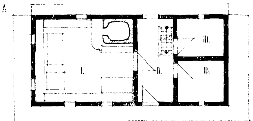
PÔDORYS PRÍZEMIA
