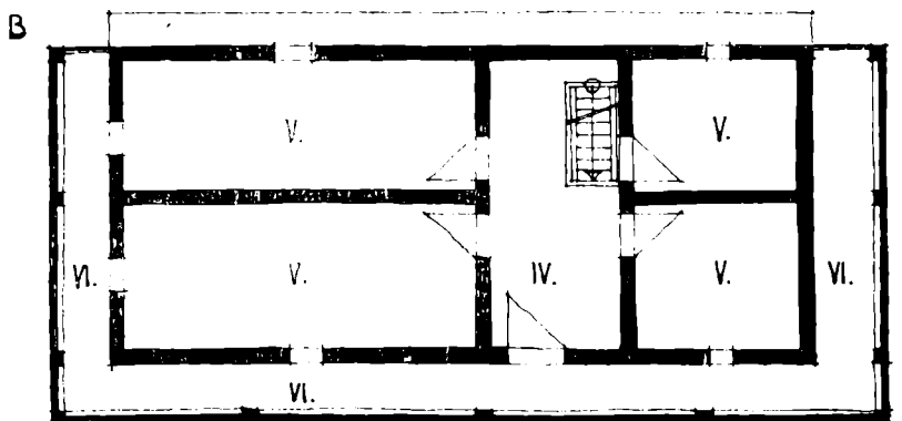
PÔDORYS 1. POSCHODIA
