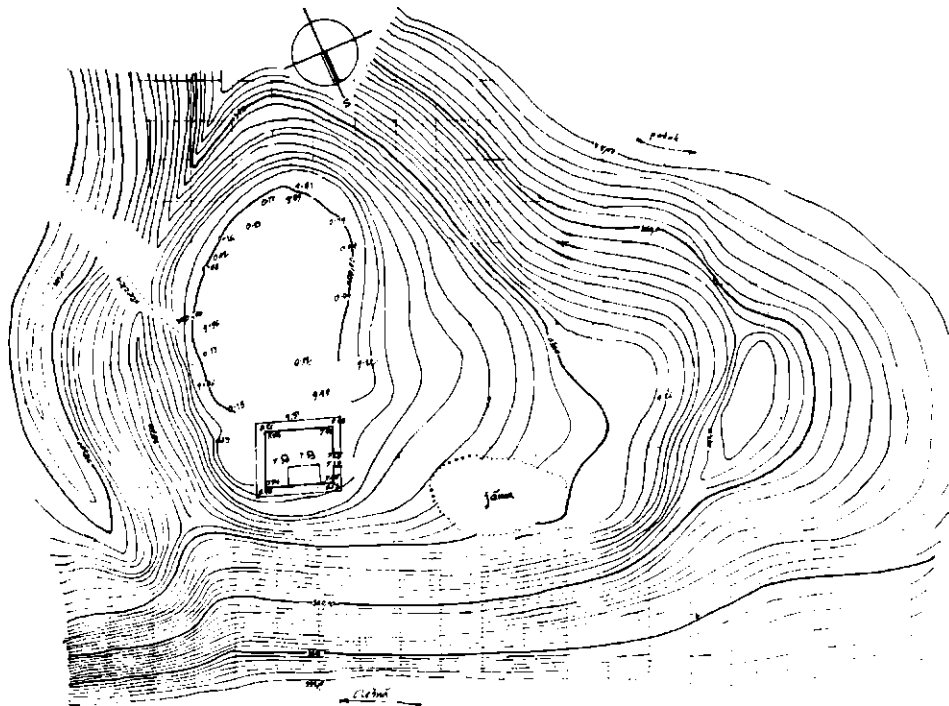
Obr. 2. DSO Liplna, pôdorysné a výškové zaměření.
