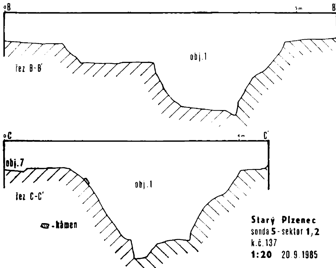
Obr. 5. Sonda 5/85. Profil zásobní jámy – sklípku. Obj. 1.
