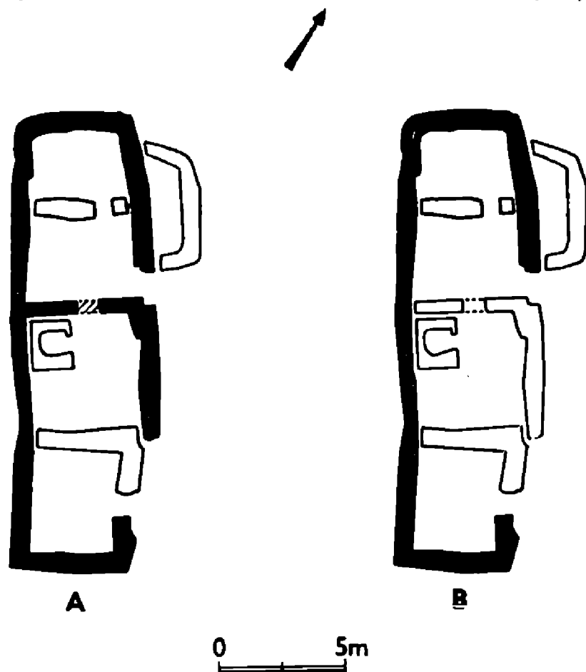
Obr. 1. ZSV Svídna (Drnek o. Kladno). Obytný dům usedlosti č. 3. A – Provázání souvislé obvodové zdi domu vymezující jeho počáteční rozsah a severní zdi jízby, patrné při preparaci v horní hladině zdiva; ostatní zdivo přisazené na spáru. B – Souvislá obvodová zeď domu vymezující jeho počáteční rozsah a přisazení severní zdi jízby (patrné v nižší hladině zdiva) a ostatního zdiva na spáru. (Souvislé provázané zdivo černě, zdivo přisazené na spáru bílé.)
