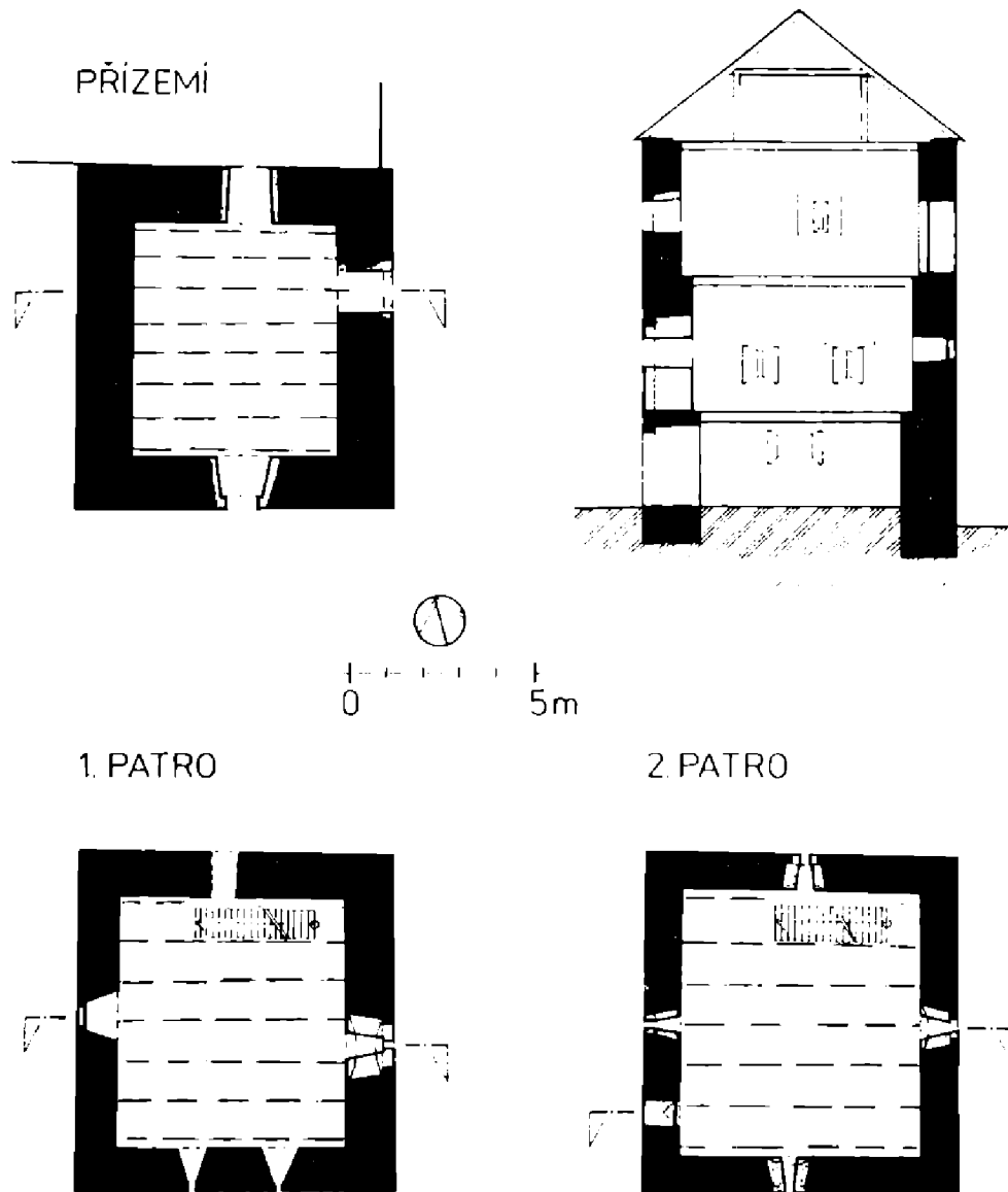
Obr. 5. Kouskova Lhotka, věž tvrže (zaměření M. Rykl a J. Úlovec 1985 až 1992).
