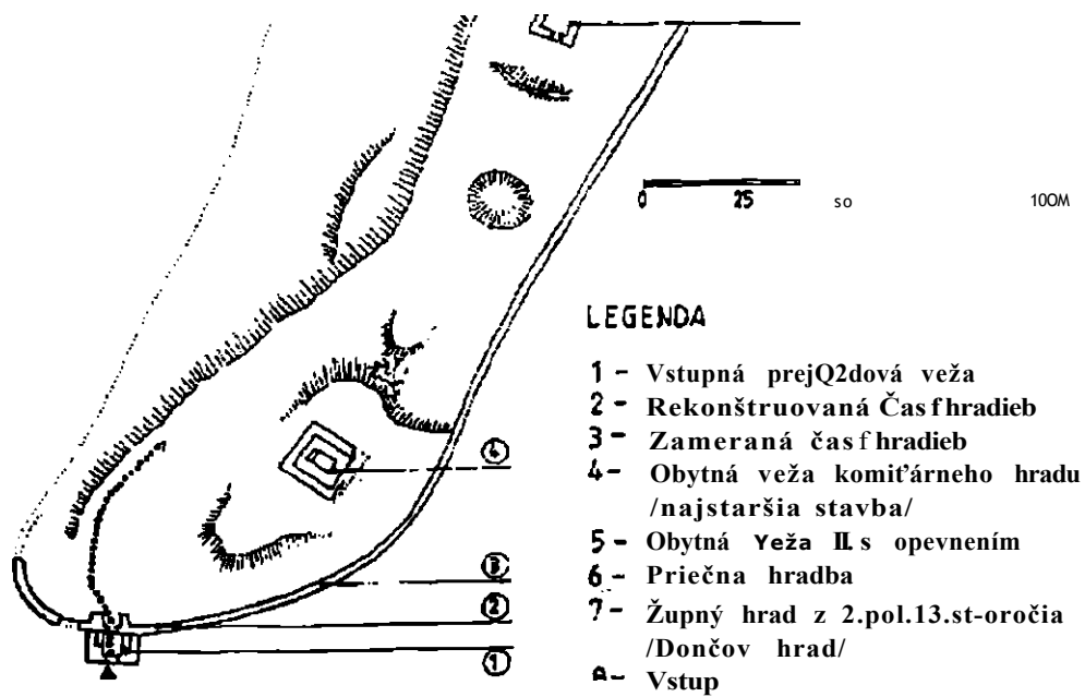
Obr. 3. Zvolen - Pustý brad. Výskumom odkrytý komitárny hrad s astou rehígia. Zamerali M. Báblk-M. Šlmkovic.
