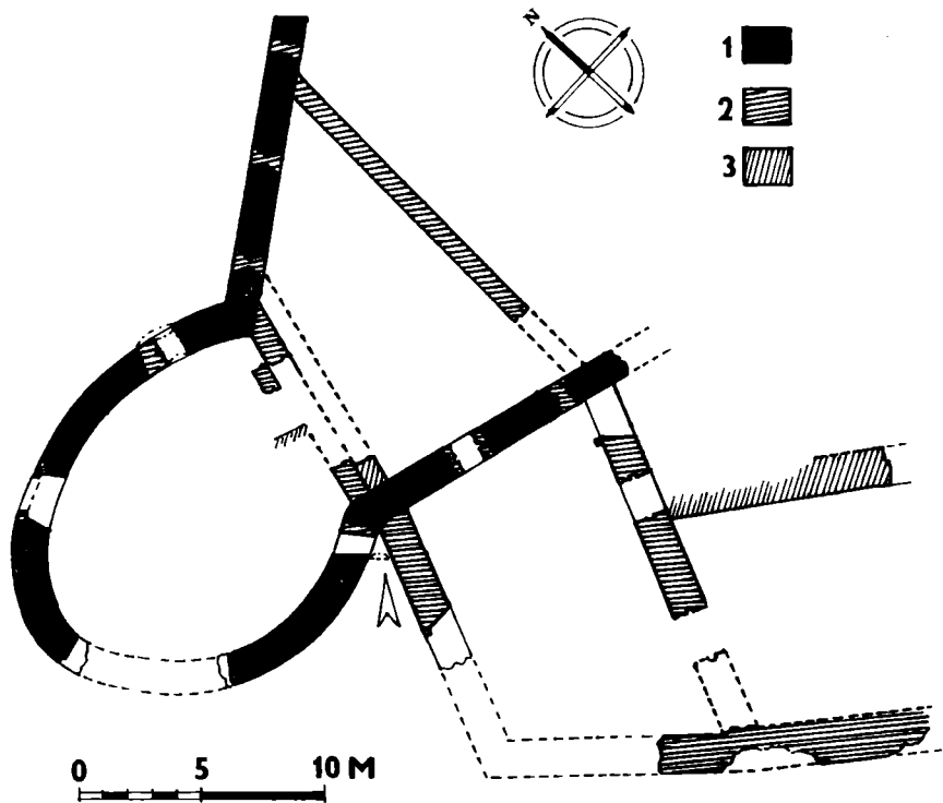
Obr. 11. Pôdorys poschodí objektov v západnej časti Oponického hradu s označným situáciou arkierového prevétu (1 – raná renesancia; 2, 3 – neskorá renesancia). Kresba autor.
