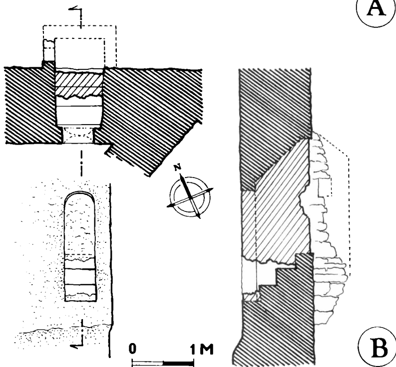
Obr. 1. A: Pódorys hradu Uhrovec s vyznačením polôh jednotlivých prevětov. Zameranie: Inž. geodézia Bratislava, kresba autor. B: Pódorys, pohľad na portálik a rezopohľad neskororománským prevetom hradu Uhrovec. Zameranie a kresba autor.
