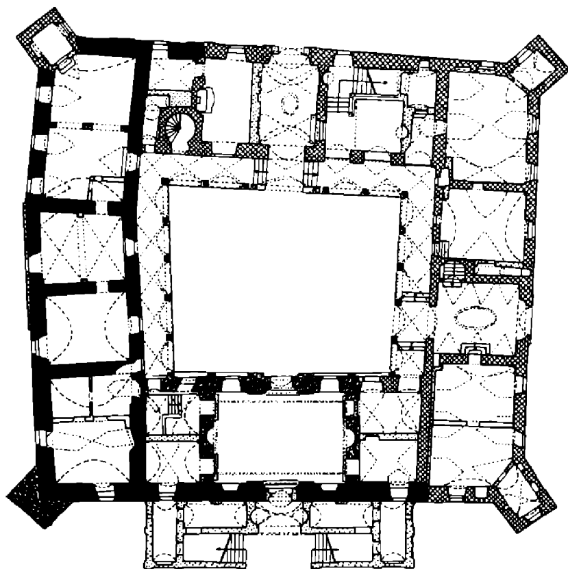
Obr. 9. Milotice, analýza přízemí zámku. Černě je vyznačeno gotické zdivo (zrněně hypoteticky), mřížkovaně renesanční, tečkovaně barokní, bíle pozdější.
