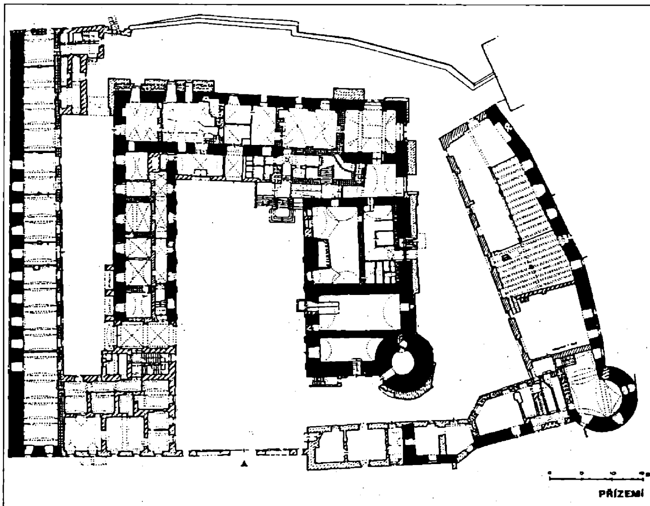
Obr. 1. Vlašim, zámek. Přízemí zámku ve stavebně historické analýze SÚRPMO: Černé zdivo gotické, mřížky kolmé na konstrukci – renesanční, šikmá šrafura – barokní, šikmé dvojčáry – klasicistní, tečkované – novodobé. Hypotetické zařazení – přerušované. Podle F. Kašičky – upraveno (jižní palác a konírna) dle nových nálezů autorkou.
