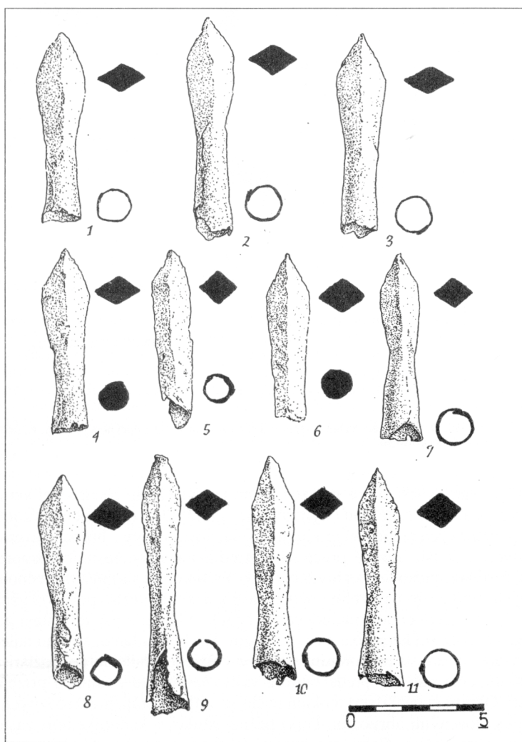
Obr. 8. Čabradský Vrbovok-Táborisko. Hroty striel z opevnenej polohy. Kreslila M. Severínová.
