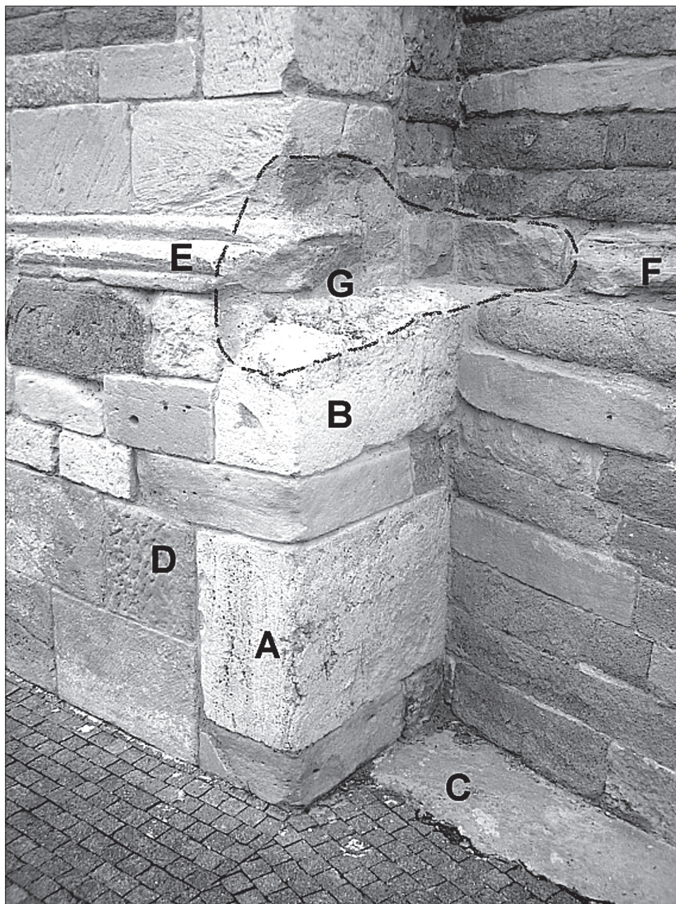
Obr. 7. Roh lode a kontakt s apsidou – sokel južnej steny Kostola sv. Emeráma. A-B: Armovacie rohové kvádre. A – pórovitý travertín, B – riasový vápenc, C – základový kameň zo sivého vápenc. D – sekundárne použitý kváder z pieskovca so špicovaným povrchom, E+F – soklová rímsa a G – silné porušenie rímsy a prilahlých kvádrov (okontúrované). V kontúre v pravej časti sú dva nové kvádre s odlišnou maltou.
