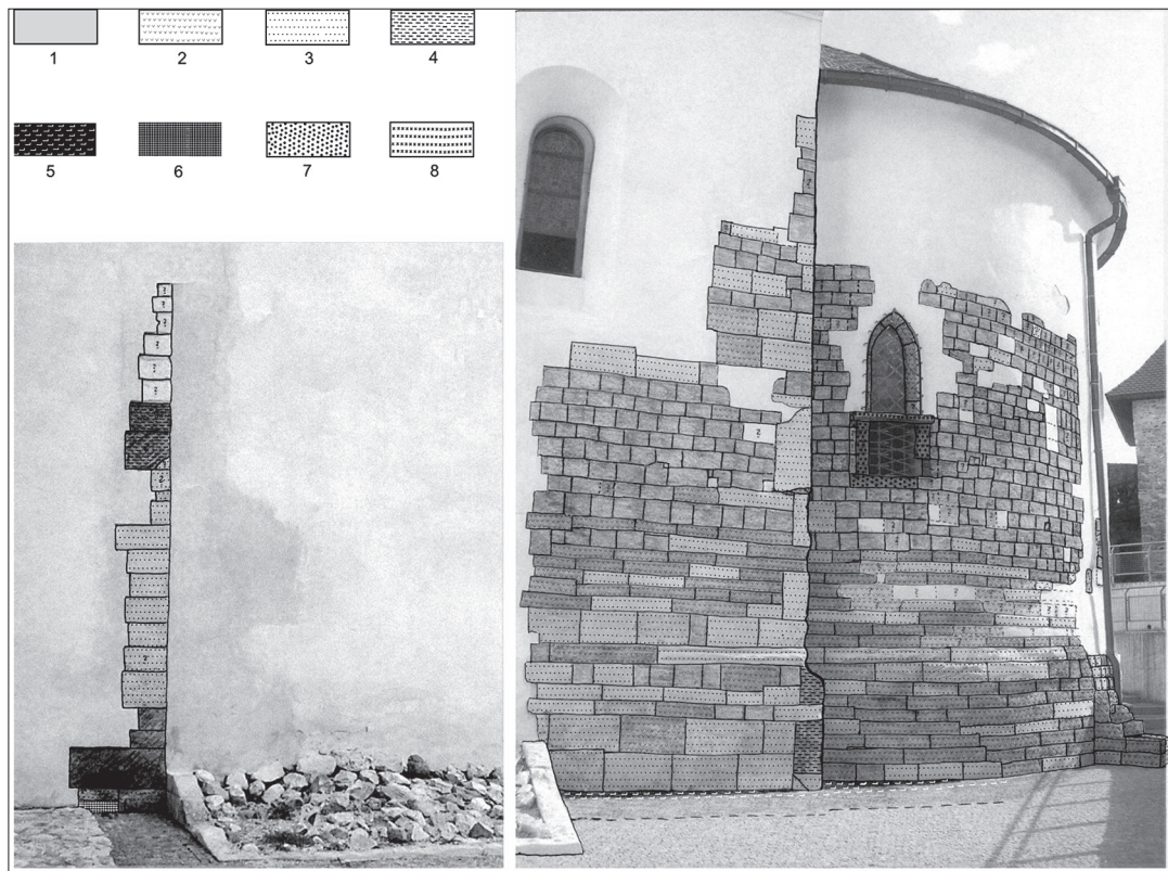
Obr. 2. Horninové zastúpenie v kvádrioch južnej steny lode a apsidy Kostola sv. Emeráma: 1 – belavý organogénny vápenec, 2 – pestrofarebné tufy, 3 – žltkasté pieskovce, 4 – travertín až riasový vápenec, 5 – tmavosivý vápenec, 6 – bordový kremenec, 7 – horický pieskovec a 8 – litavský vápenec. Vľavo je roh staršieho kostola zvýraznený armovacími kameňmi. Pôvodne sú len 4 kamene.
