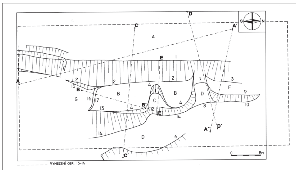
Obr. 5. Púdorys povrchového tvaru obj. 1.
