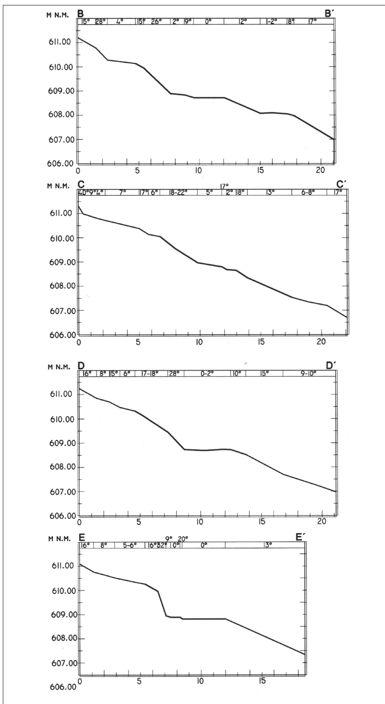
Obr. 12. Profilové křivky povrchového tvaru obj. 10. Abb. 12. Profilkurve der Oberflächenform von Obj. 10.
