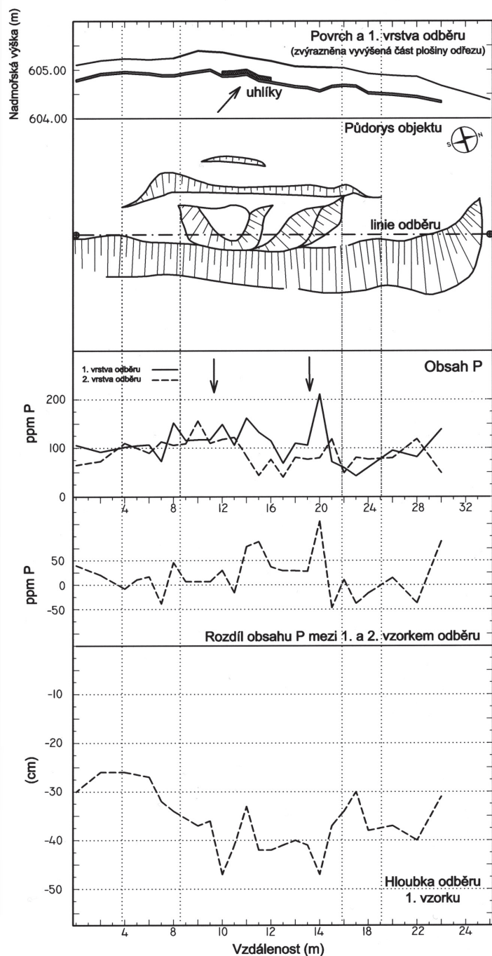
Obr. 18. Znárodnění půdorysu obj. 10, míst odběru a výsledků fosforečnanových analýz.
