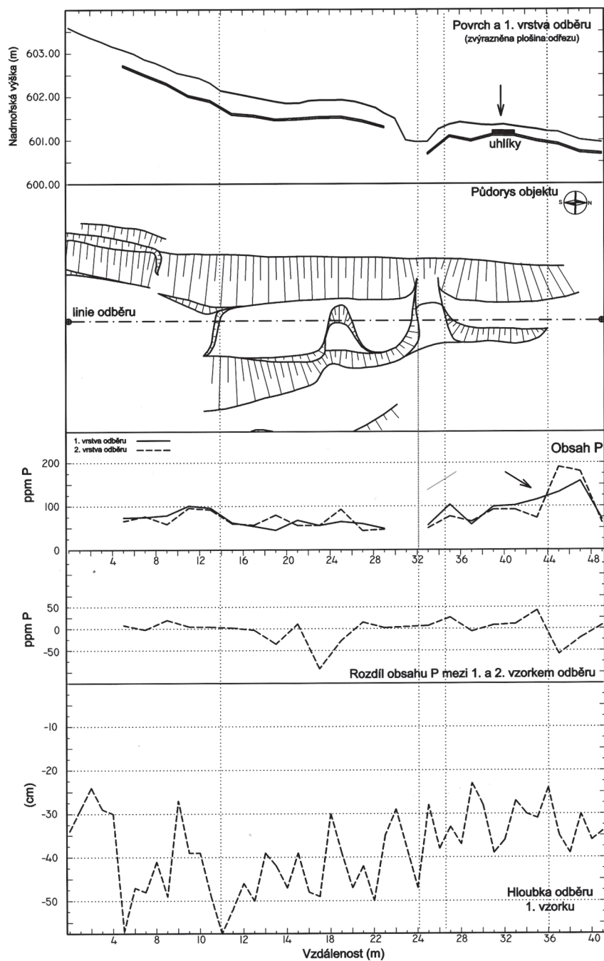
Obr. 14. Znázornění půdorysu obj. 1, míst odběru a výsledků fosforečnanových analýz (2. linie).
