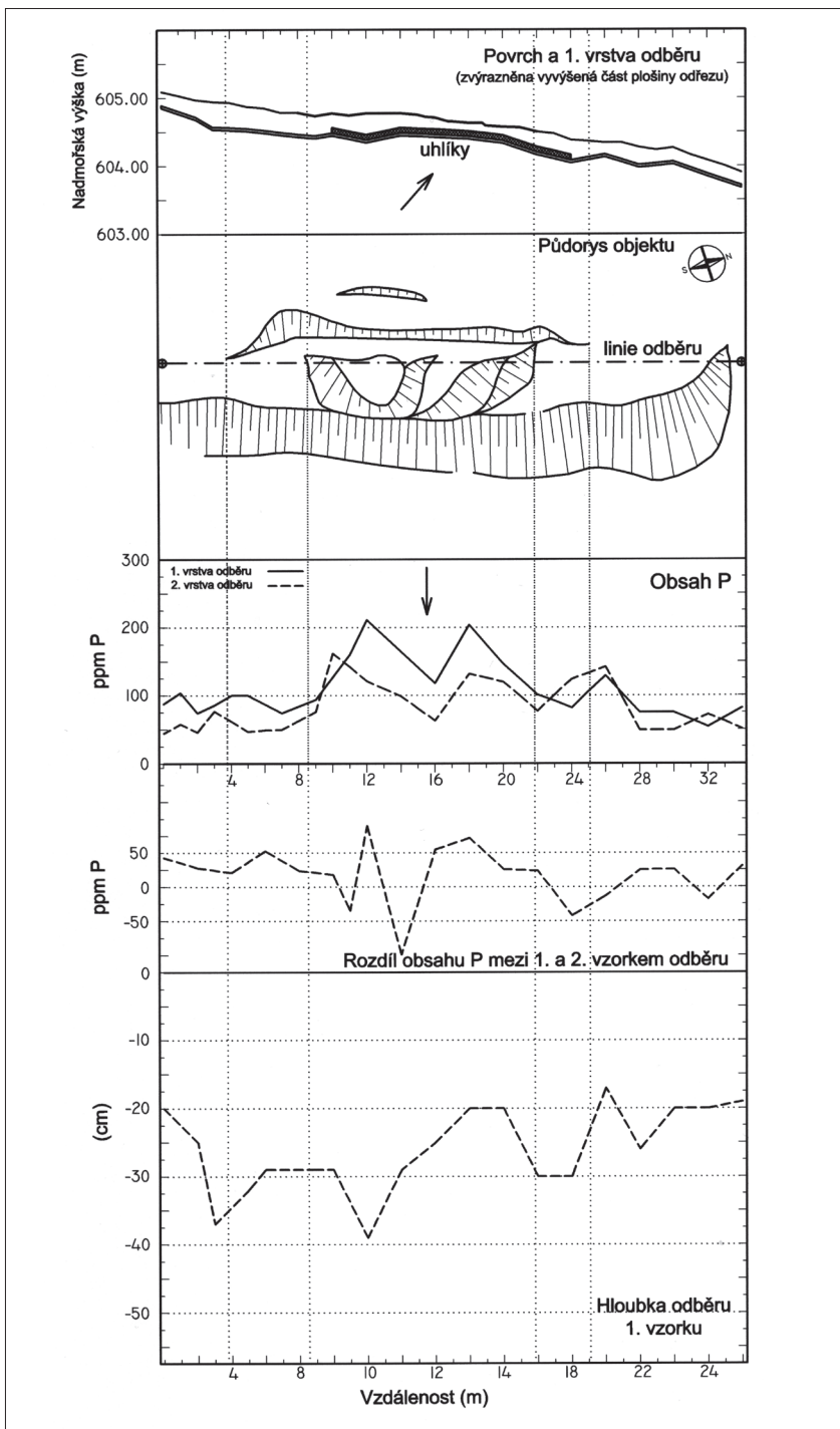
Obr. 17. Znázornění půdorysu obj. 6, míst odběru a výsledků fosforečnanových analýz (2. linie).
