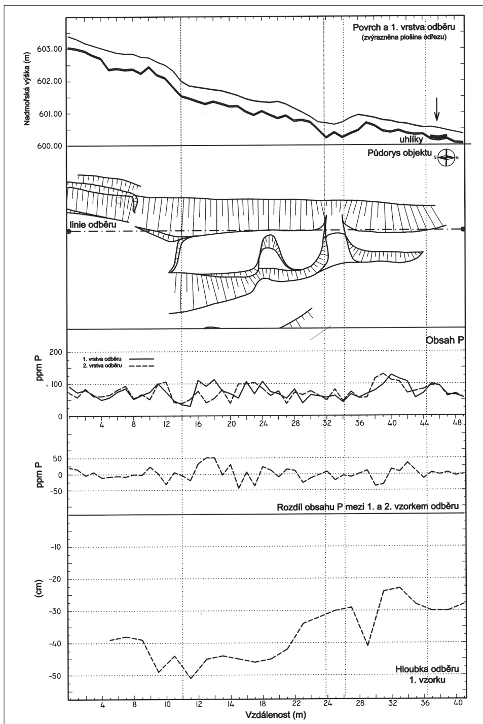
Obr. 13. Znáznornění půdorysu obj. 1, míst odběru a výsledků fosforečnanových analýz (1. linie).
