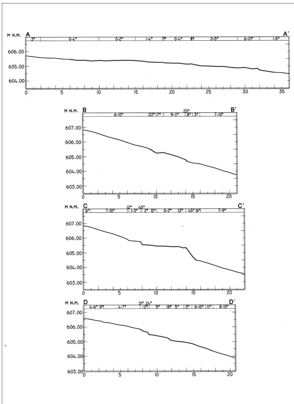
Obr. 10. Profilové křivky povrchového tvaru obj. 6.
