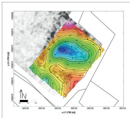
Obr. 7. Výsledok mikrogravimetrických meraní – izočíary hodnôt neúplných Bouguerových anomálií pre korekčnú hustotu 2,0 \text{ g.cm}^{-3} . Ako spodná vrstva obrázku sa nachádza horizontálny amplitúdový rez pre hĺbku prieniku 125 cm. Plné čierne krúžky zobrazujú polohy mikrogravimetrických bodov.
