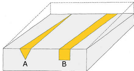
Obr. 13. Rozdíl v profilu rýh při inkrustaci za horka (A) a při tautzii, tj. inkrustaci za studena (B). Při odebrání povrchu předmětu obroušením či korozi dochází v případě A k zužování původní linky, v případě B nikoli.
