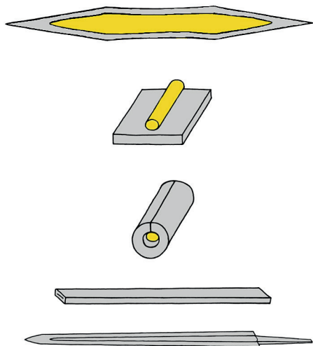
Obr. 9. Metallografickým průřezem zjištěná konstrukce čepelí (příčný řez: bílá ocel, žlutá železo) a rekonstruovaný postup její výroby.
