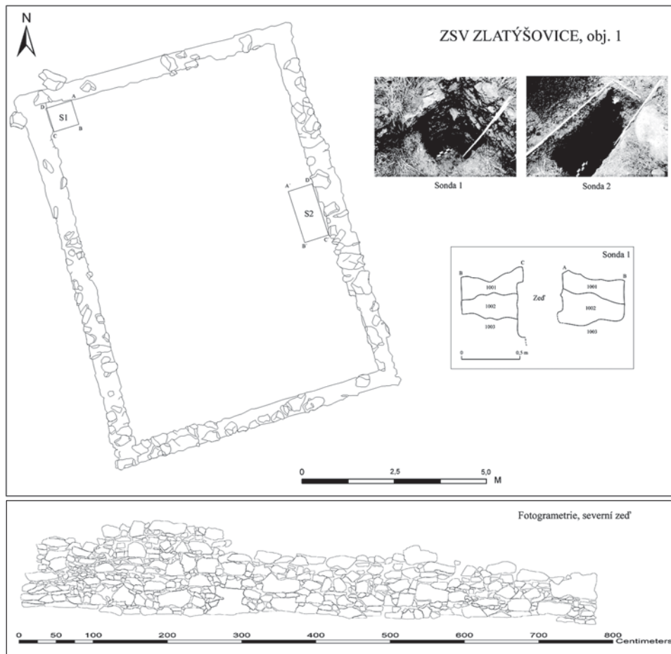
Obr. 11. ZSV Zlatýšovice (okr. České Budějovice). Půdorys kamenné stavby s polohou archeologických sond. Fotogrametrie jižní zdi. Zaměření a kresba autor.
