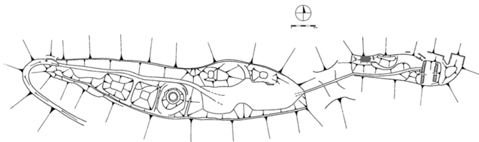
Obr. 1. Hrad Žampach, okr. Ústí nad Orlicí. Plán hradu se zakreslením sondy E. Zaměření M. Cejlová, P. Cejp.
