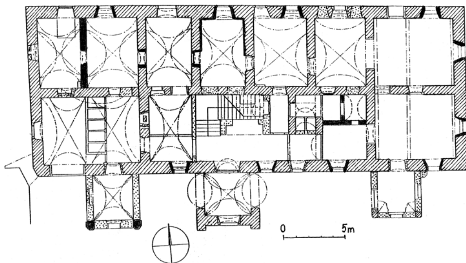
Obr. 3. Zámeček, analýza půdorysu přízemí. Šrafované – pozdně renesanční zdivo, černě je položeno zdivo barokní, tečkovaně zdivo z 19. století, bílé je zdivo 20. století. Vypracoval autor; podklad Státní projektový ústav obchodu Brno, upravené zaměření stávajícího stavu, únor 1989.
