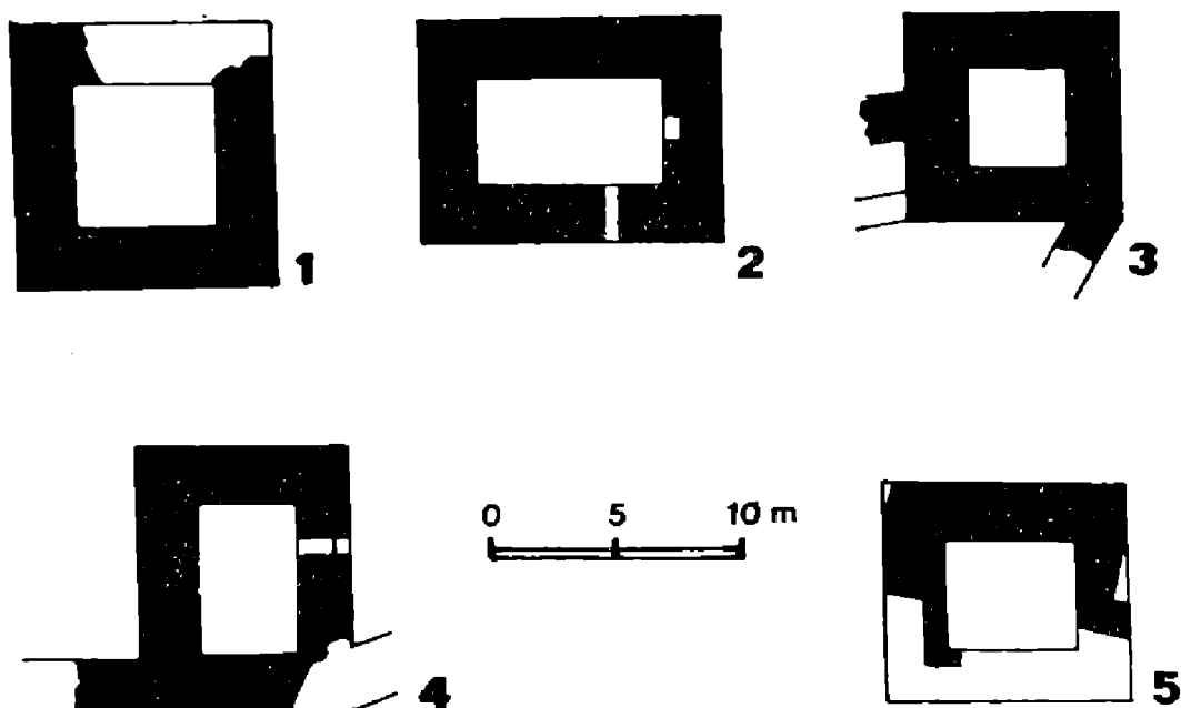
Obr. 5. Výběr z obytných věží českých hradů složitějších dispozic. 14. století. 1 – Křivkava, 2 – Kozi Hrádek, 3 – Rabštejnec, 4 – Strádov, 5 – Bradlo. 1-4 dle D. Menclové, 5 podle A. Hejny. Kresba J. Zikové.
