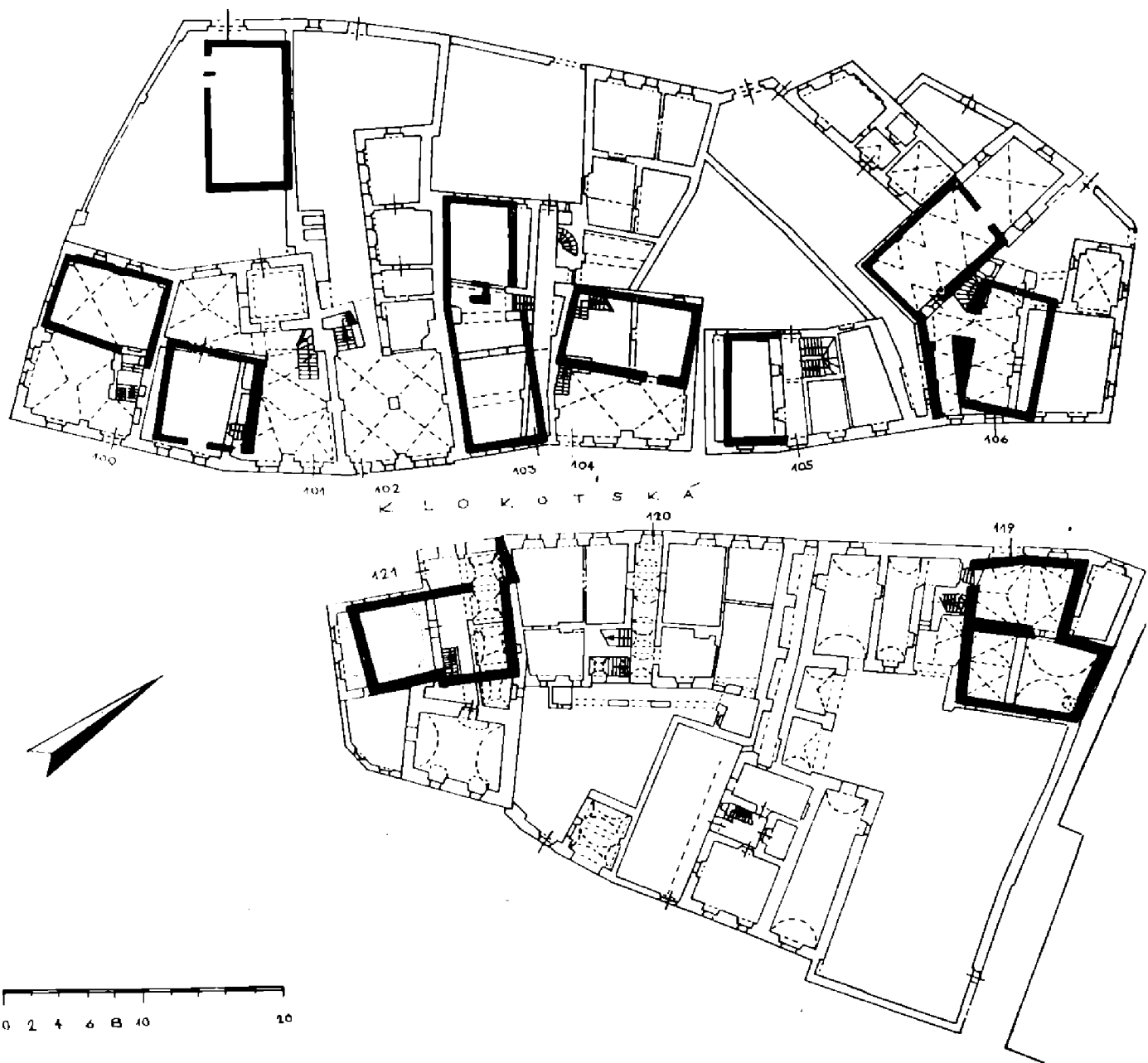
Obr. 1. Tábor. Domy v Klokočské ulici. Přizemí se zakreslením situace gotických sklepů.
