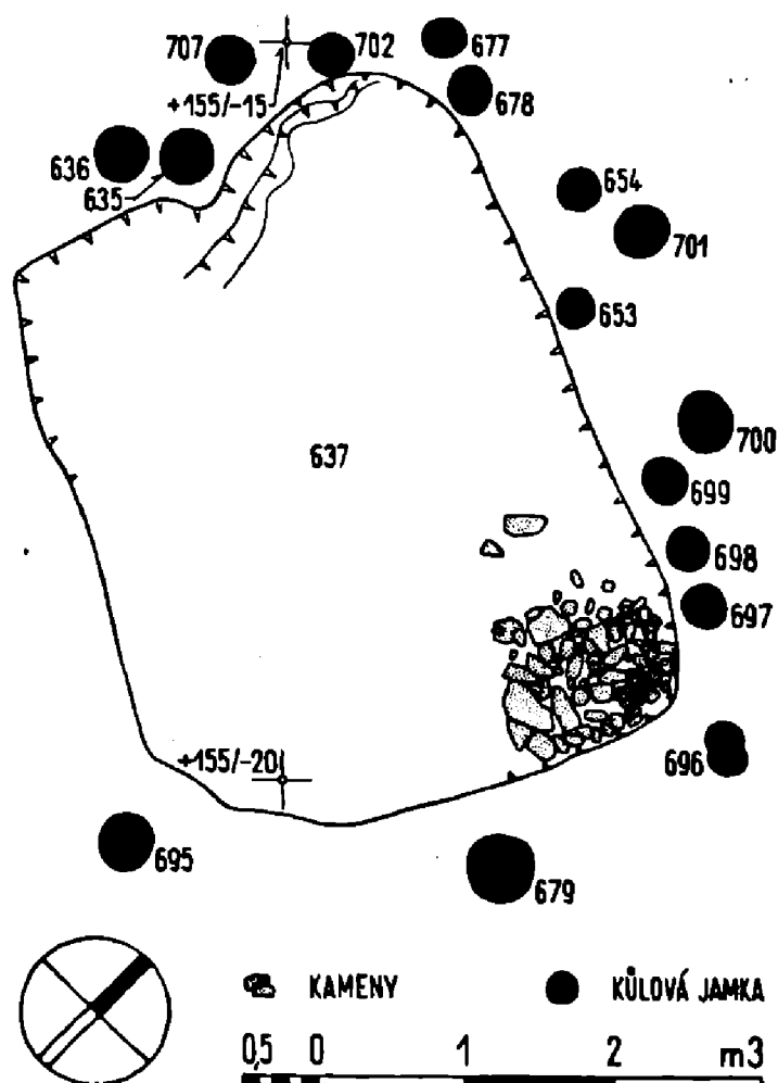
Obr. 10. Mstěnice. Zaniklá středověká osada. Půdorys chaty 637.
