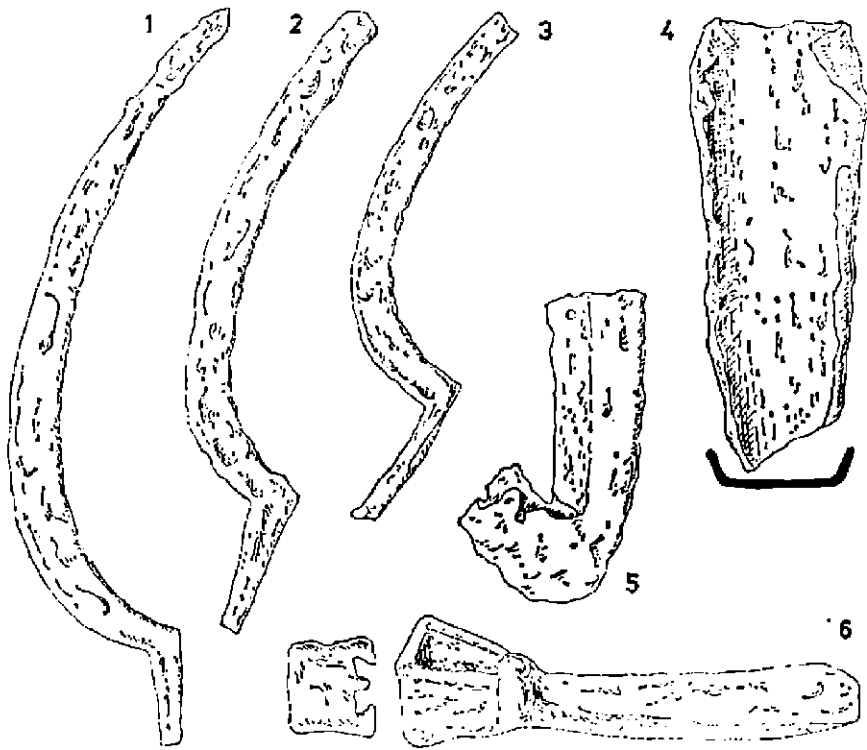
Obr. 2. Výber kováckych výrobkov zo zaniknutej stredovekej dediny Zalužany-Nemešany, okr. Spišská Nová Ves.
