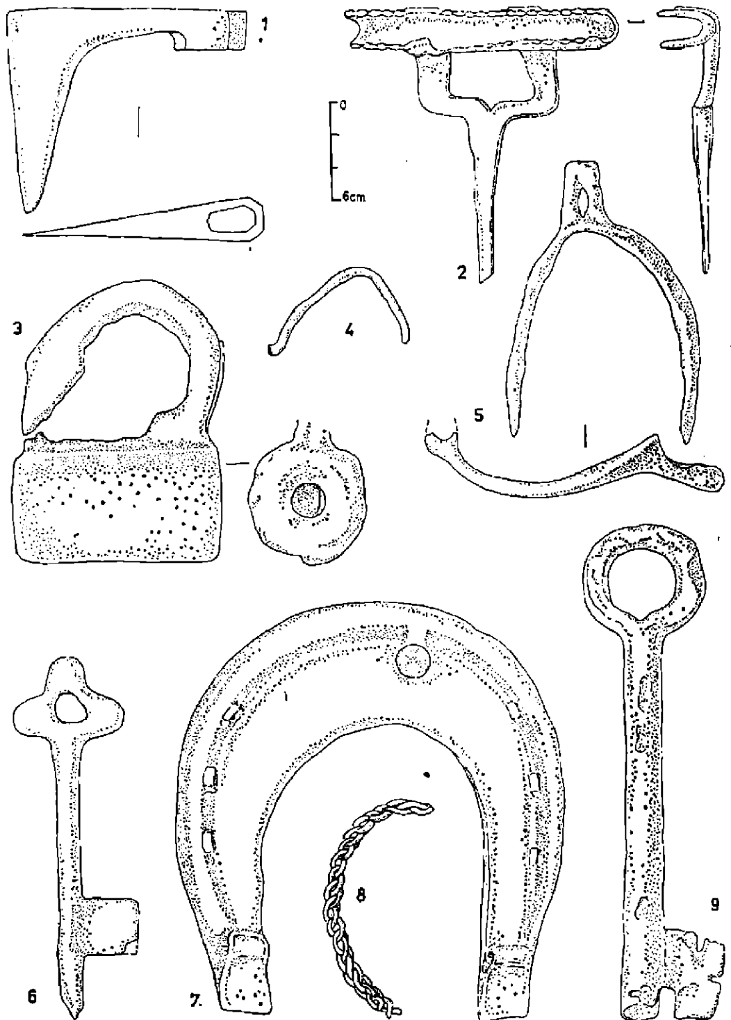
Obr. 8. Výber kováčskych výrobkov a jednoduchých ľudových ozdôb zo zaniknutej stredovekej dediny vo Svidnici, okr. Košice-vidiek.
