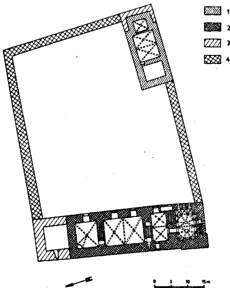
Obr. 12. Horšovský Týn hrad, okr. Domailke. Částečná rekonstrukce patra hradu. 1—1. raněgotická fáze; 2—2. raněgotická fáze; 3—3. raněgotická fáze; 4—4. raněgotická fáze. Kresba J. Minarčíková.
