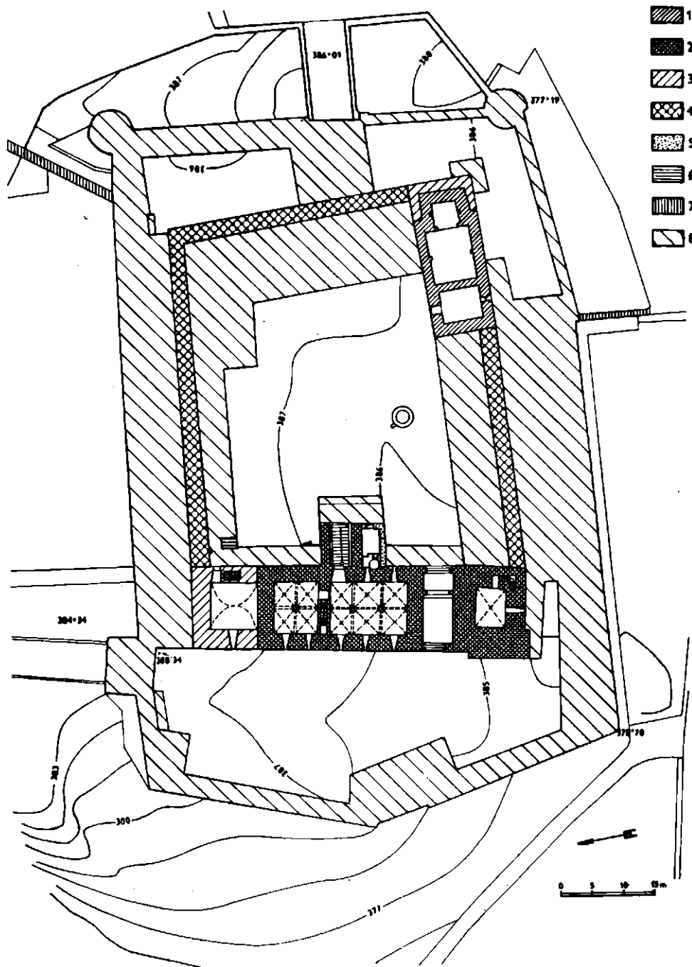
Obr. 11. Horšovský Týn hrad, okr. Domažlic*. Částečná rekonstrukce přízemí hradu zakreslená do obrysu dnešního zámku. 1 — 1. raněgotická fáze; 2 — 2. ranogotická fáze; 3 — 3. ranogotická fáze; 4 — 4. raněgotická fáze; 5 — pozdnegotické zdivo; 6 — blíže nedatované gotické zdivo; 7 — pozdnegotické městské hradby; 8 — renesanční a mladší. Kresba J. Minářčiková.
