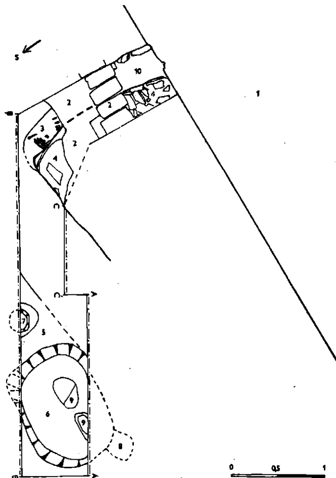
Obr. 4. Horšovský Týn hrad, okr. Domažlice. Situace sond 1-3. 1 — nádvoří zeď starší kaple; 2 — recení stavební zásahy, 3 — zjištěná část hrobové jámy; 4 — předzáklad patrně renesančního zdiva; 5 — zahloubený objekt; 6 — jáma v jeho dně; 7, 8—kulové jámy 1 a 2; 9—ztrouchnivělé želevo; 10 maltová vrstva. Kresba L. Krušinová.
