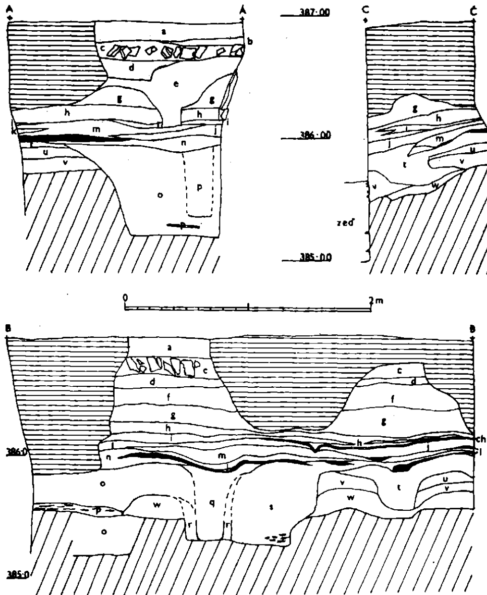
Obr. 5. Horiiovský Týn hrad, okr. Domažlice. Profily A, B, C v sondách 1-3. Popis vrstev: a - žluté písčité; b - šedozelená sypká kamenitá; c - tmavěhnědé hlinité lůžko dlažby; d - světlá sypká s maltou a kameny; e - hnědá sypká s maltou, kameny a zlomky cihel; f - tmavě hnědá sypká kamenitá; g - tmavěšedá kamenitohlinitá; h - bílá tuhá maltová masy s kamenitou mezlvrstvou; ch - jemná rezavá; i - kamenitá s pískem; j - jedá kompaktní jílovitopísčité; k - světlá písčité; l - propálená mazanice; m - kamenitá; n - zelenorezavá tuhá promíjená jílovitá s kameny a uhlíkatými propásty; o - měkká jílovitá promíjená se stopami ztrouchnivělého dřeva; p - ztrouchnivělé dřevo (kul. 2 v profilu A v průmětu); q - jedá mokrá hlinitá se zbytky dřeva; r - šedá mokrá hlinitá s uhlíky; s - šedozelená mokrá hlinitá; t - promíjená měkká jílovitá s uhlíky a ztrouchnivělým dřevem; u - promíjená měkká jílovitá s oblázky; v - šedá jílovitá s uhlíky; w - zelenavá jílovitá. Černé uhlíky, vodorovně šrafovány recentní zásahy, šikmo jílovité položí. Kresba L. Krušinová, T. Durdík.
