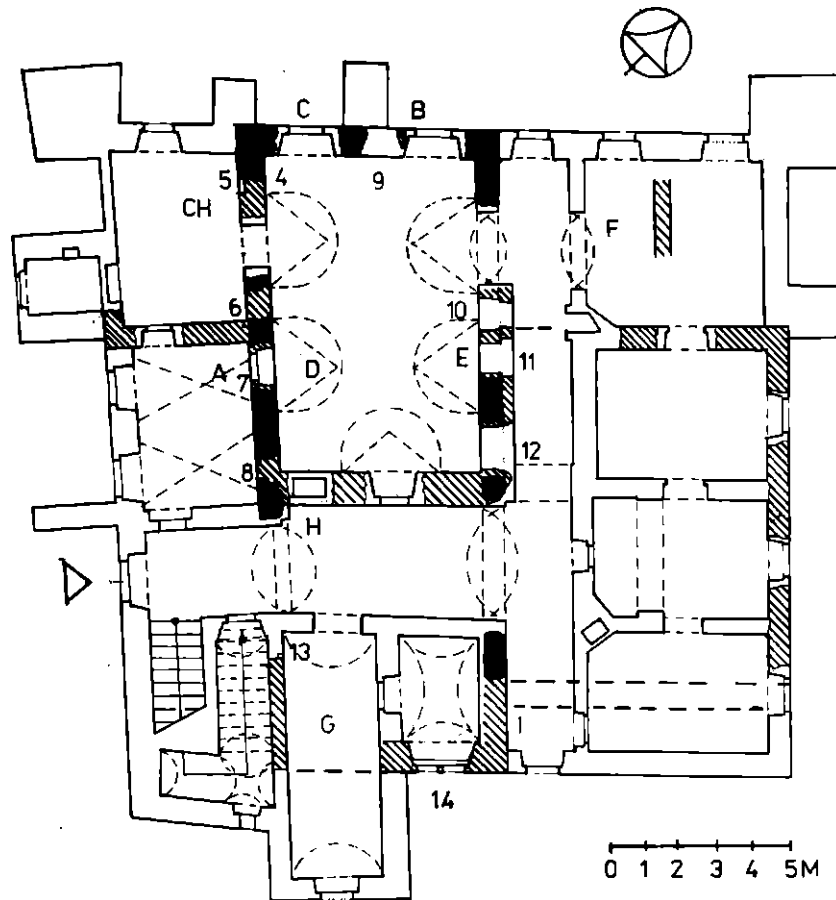
Obr. 3. Bratislava — Devín, kaštieľ na Hutníckej ul. C. 25. Pôdorys prízemnia, stavebná historická analýza. Clerne mŕtvo I. etapy, šrafované murivo II. a III. etapy, 4. ostienle okna z I. etapy. 5. okno z III. etapy, 6. otvor z II. etapy. 7. portál z III. etapy. 8. vetrací otvor z I. etapy. 9 a 12. otvory z III. etapy. 13. portál z III. etapy. 14. okno s paspartou z III. etapy. Písmenami A—H sú označené archeologické sondy.
