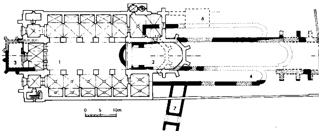
Obr. 1. Půdorys kostela sv. Petra a Pavla na Vyšehradě na základě výsledku archeologických výzkumů: černě značené – zaniklé středověké zdivo známé nebo zjištěné archeologicky (včetně zdiva zjištěného v negativu), šikmá šrafura – dotvořený průběh zdiva mezi sondami, 1 – půdorys dnešního kostela, 2 – pozdně gotický, případně renesanční kostelní závěr, zbořený při regotizaci J. Mockerem (1885–1887), 3 – zaniklá gotická síň před západním čelem kostela, 4 – apsida románské jižní lodě, 5 – závěr kostela ze 14. století, 6 – situace bývalé zvonice, 7 – románský most, spojující kostel s knížecí a královskou akropolí.
