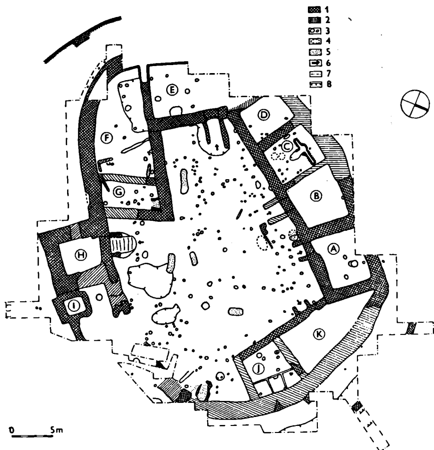
Obr. 2. Lelekovice-hrad. Celkový plán výzkumu vnitřního hradu (1984—1990). 1 — dochované zdivo, 2 — zdivo v negativu, 3 — křivé jamky, 4 — nejisté zahloubení, 5 — propáleno, 6 — vchod, 7 — hranice výzkumu, 8 — zahloubení.
