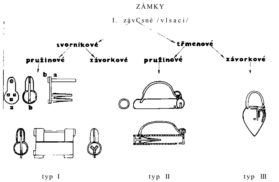
Obr. 7. Třídění a typologické schéma vrcholní středověkých závěsných zámků podle nálezů z Táborská.
