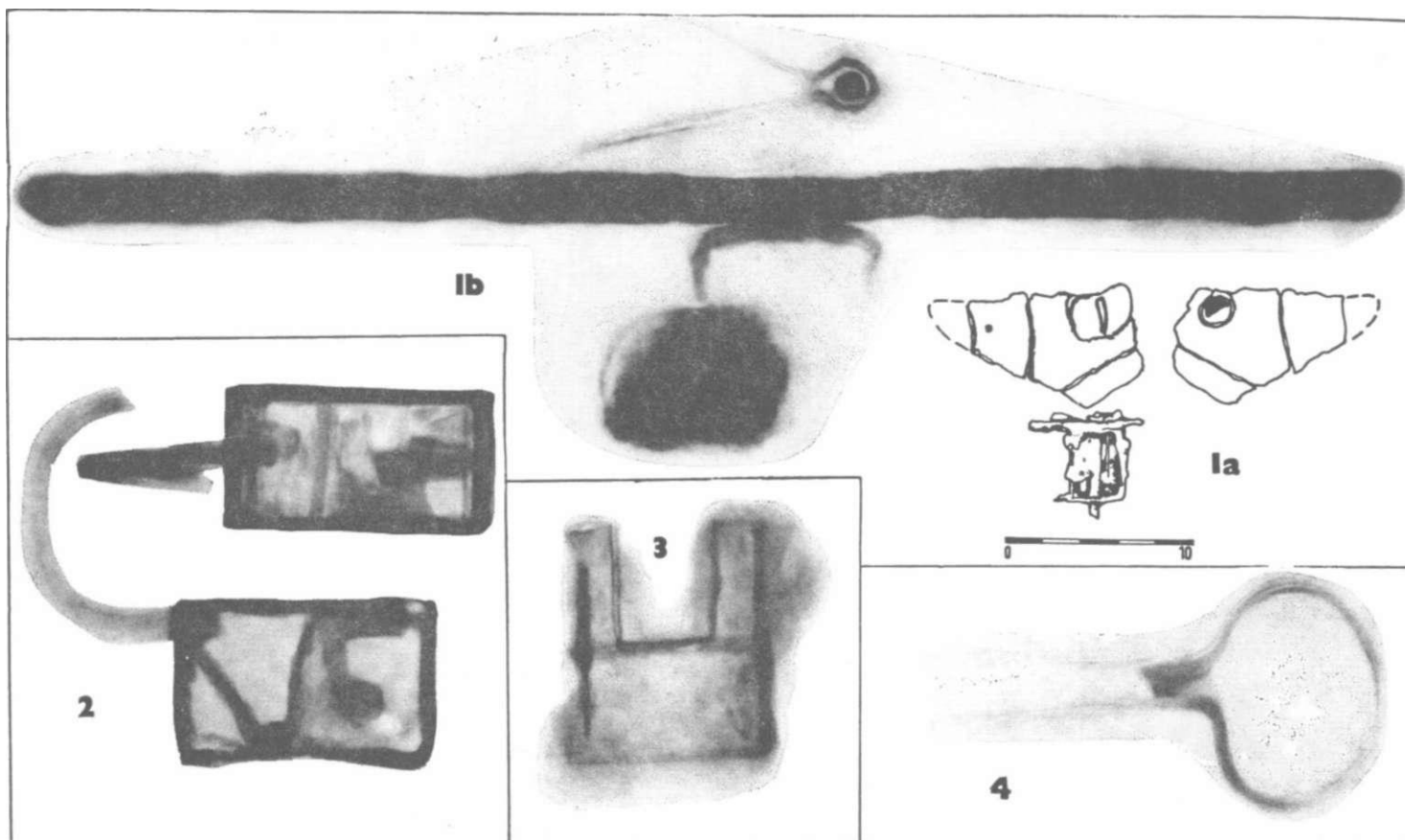
Obr. 18. Stavební kování (Sezlmovo Ústí, Kravín 1): 1a: trojúhelníkový krycí štít a zámková skříň nepřenosného zámku typu IVbj 1b: rentgenový snímek tíhož exempláře s dobře zachovalou zámkovou skříň, nad níž je pásová závera typu I s přitlačnou pružinou; 2: rentgenový snímek vnitřní konstrukce závěsného zámku třmenového závorkového; 3: rentgenový snímek závěsného zámku svorníkového pružinového s vyjmutým svorníkem; 4: rentgenový snímek otočného klíče typu X s patrnou konstrukcí oka (volný konec zasunut do dutiny dřívku).
