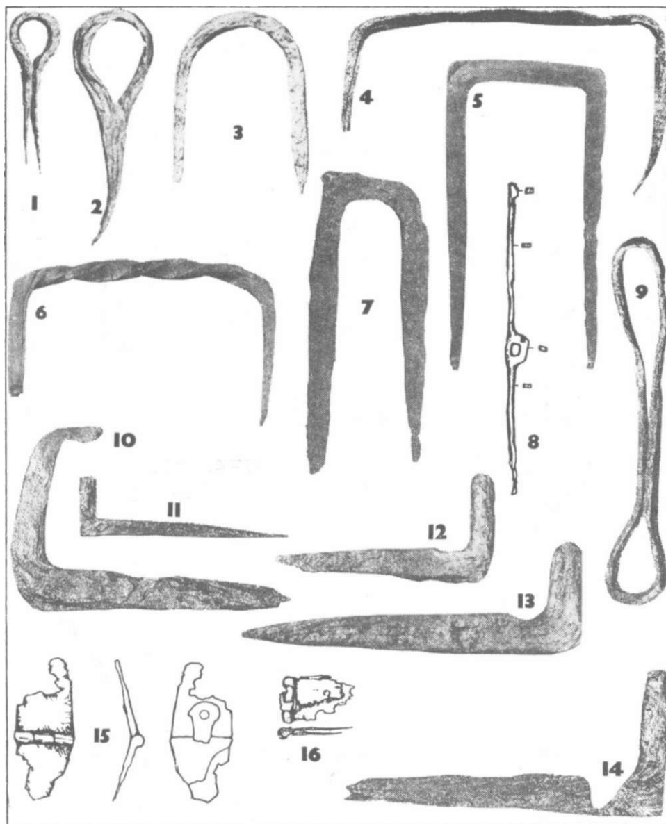
Obr. 12. Stavební kování (Sezlmo Ústí): 1—2: oka s trny; 3—7: skoby dvouramenné; 8: kotva řetězu; osmlckovltá petlice; 10—14: skoby jednoramenné; 15—16: kloubové panty.
