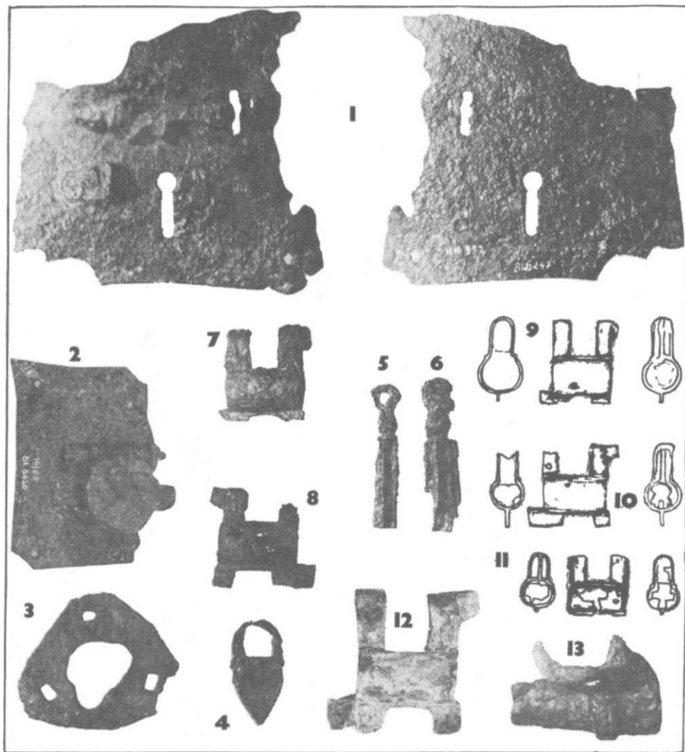
Obr. 14. Stavební kování (Sezlomovo Ústí, staré šbirkové fondy Muzea HRH Tábor): 1—2: nepřenosné zámky typu IVa; 3: kování klíčového otvoru; 4: zámek závěsný třmenový; 5—6: závorkový; zásuvné klíce s lamelami; 7—12: zámky závěsné svorníkové pružinové; 13: zámek závěsný třmenový pružinový.
