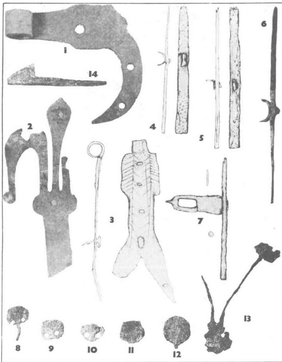
Obr. 13. Stavební kování (Sezlmo Ústí, Koží Hrádek): 1—3: panty—závěsy; 4—6: závory typu I; 7: petlco- vá závora; 8—13: části svodů; 14: zámková skoba.
