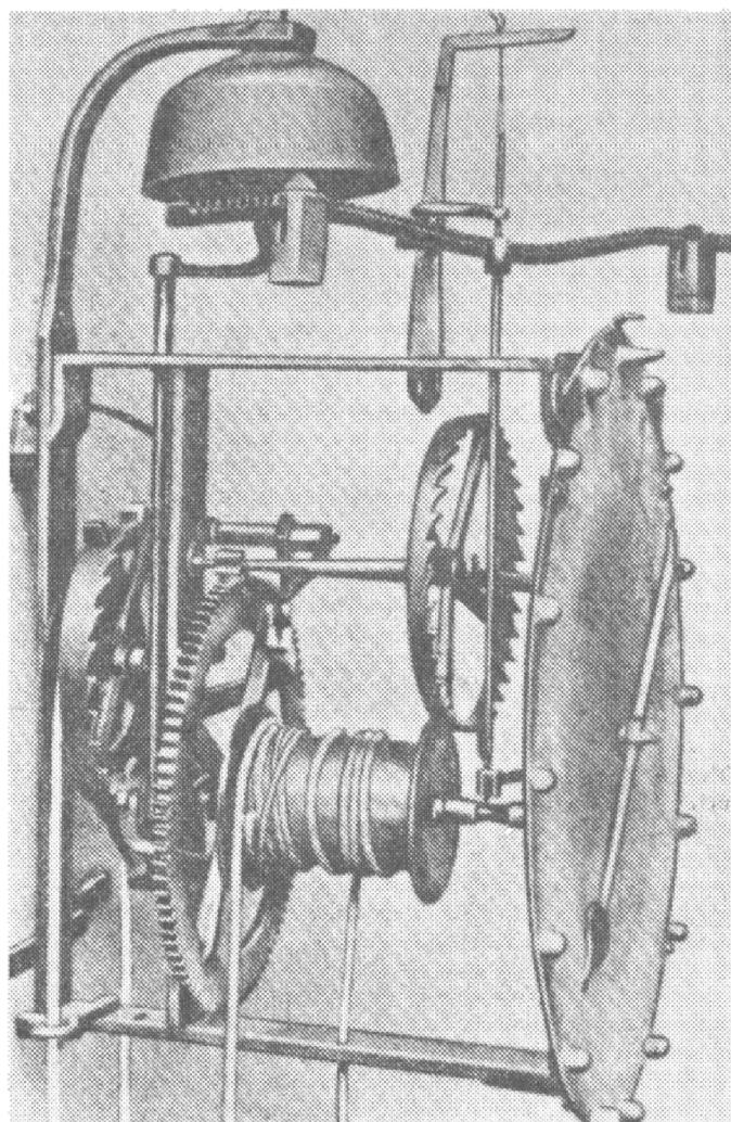
Obr. 8. Železné nástěnné zvonící hodiny ze 14.—15. století. Reprofoto H. Toušková.
