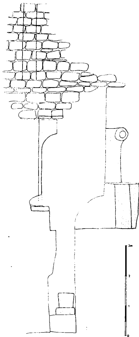
Obr. 3. Hrad Valdštejn, pohled na vchod mladší stavební podoby 3. skalního bloku. Tečkovaním lemovaná linka — sekáním upravená skála, tečkované plochy — vzdálenější pohledové plány. Měříl F. Gabriel, kresba P. Macek.
